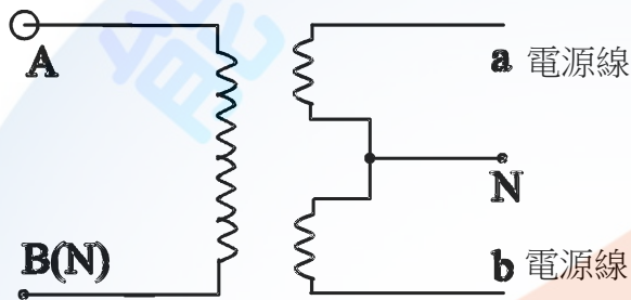
圖 1 單相三線 110/220 伏特
