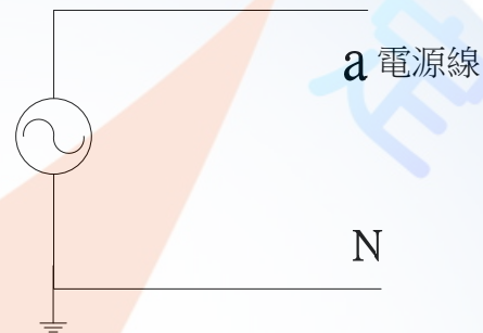
圖 2 單相二線 220 伏特
