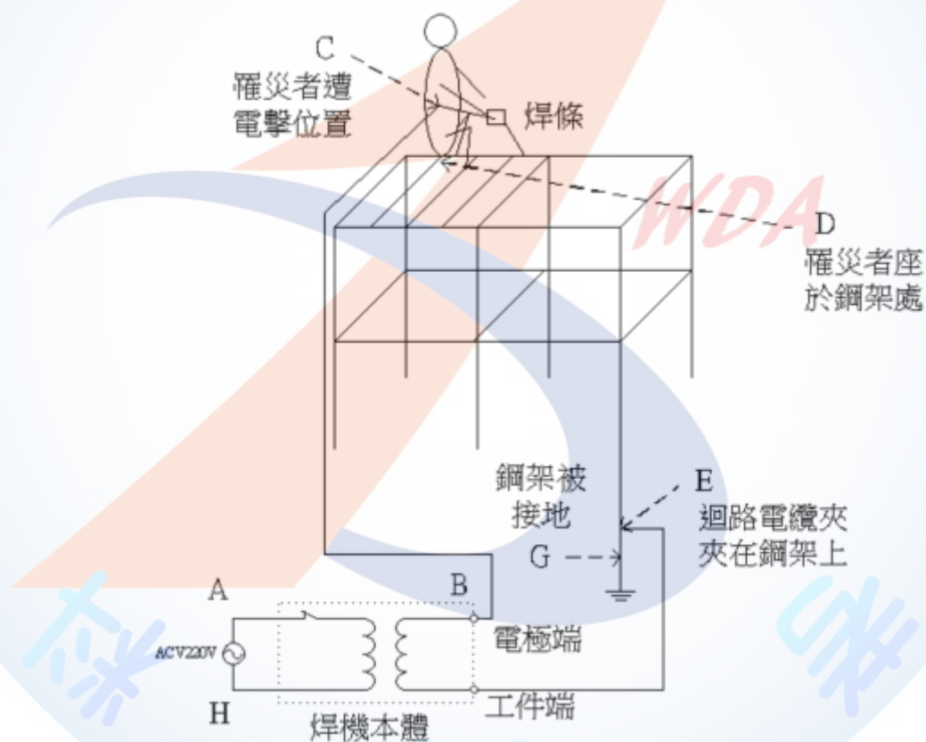
圖 罹災者於鋼架上從事電焊作業引起感電災害示意
