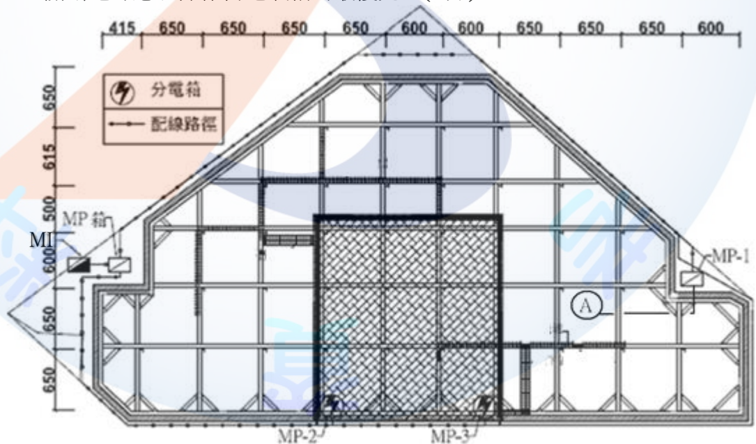
圖 某營造工地電氣箱、配線路徑示意
