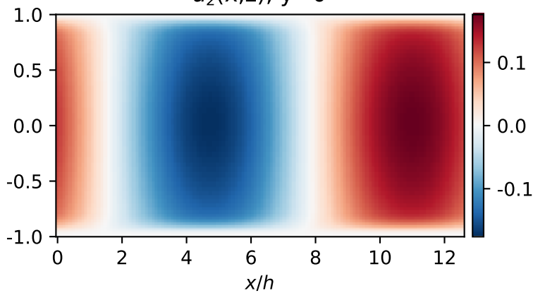
u_z(x,z), y=0
