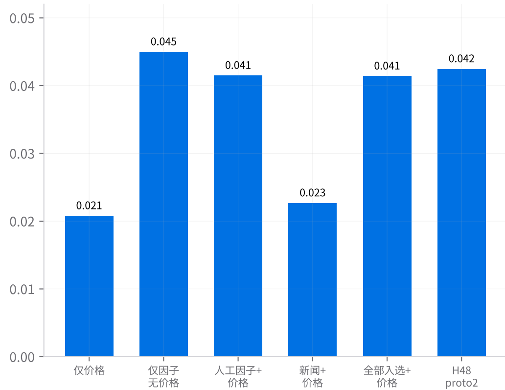
留出期 RankIC
