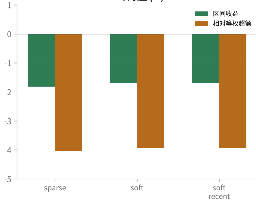
11 日收益 (%)
