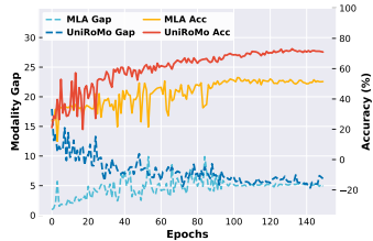
(d) Hybrid: Alternating
