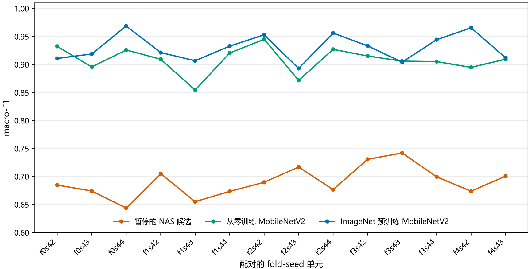
中期配对 macro-F1 (NAS 14/15, 仅诊断)
