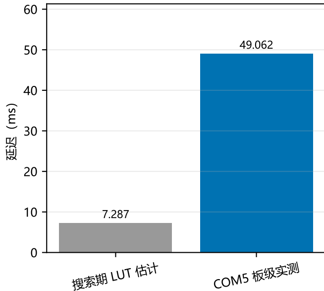
代理与板级延迟 (6.73x)
