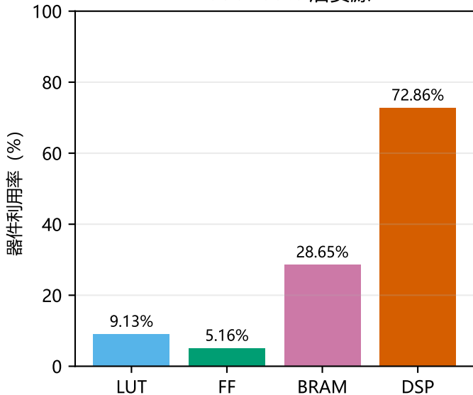
Vivado route 后资源
