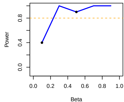
15777_G&gt;C, FB
