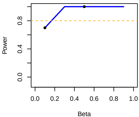
15777_G&gt;C, TC
