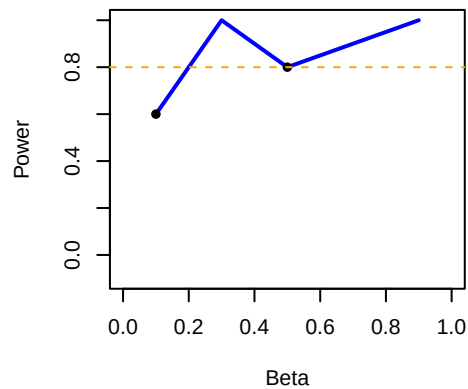
15777_G&gt;C, NS
