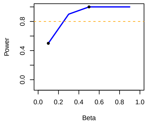
15777_G&gt;C, IM
