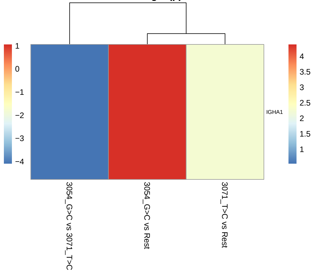
IM - -\log_{10}(p)
