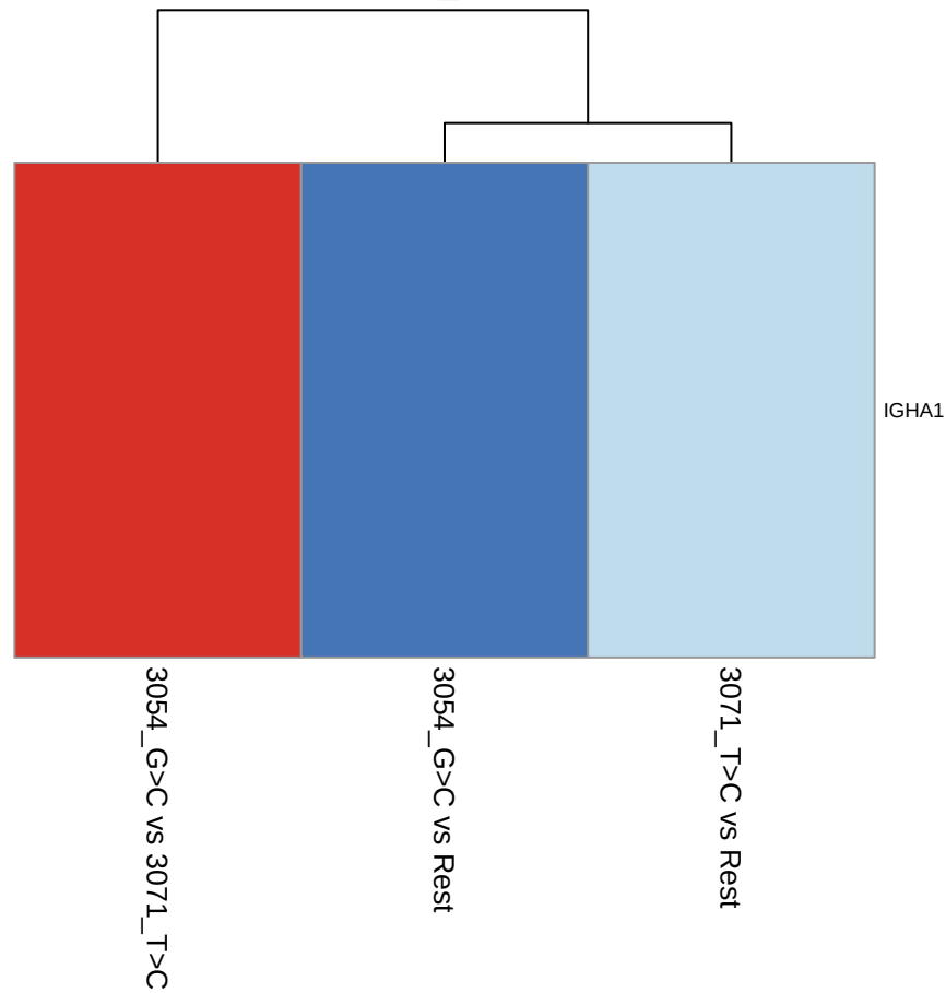
IM - test_statistic
