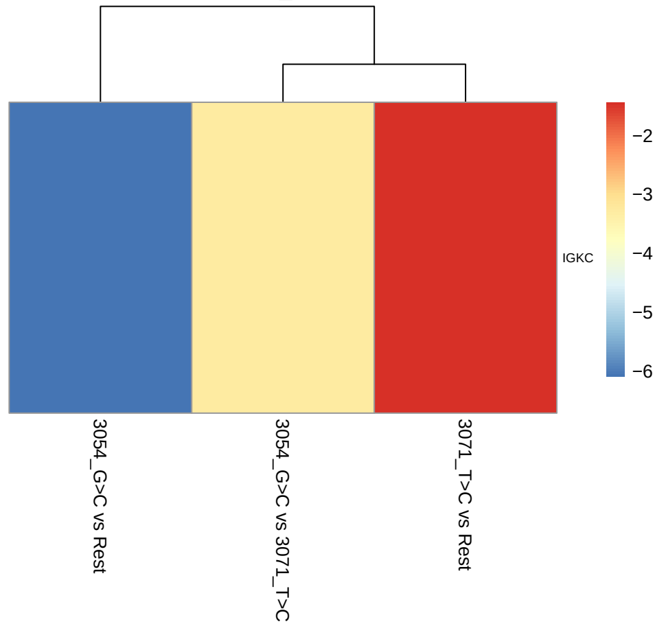
IM - test_statistic
