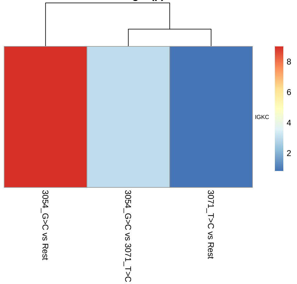
IM - -\log_{10}(p)
