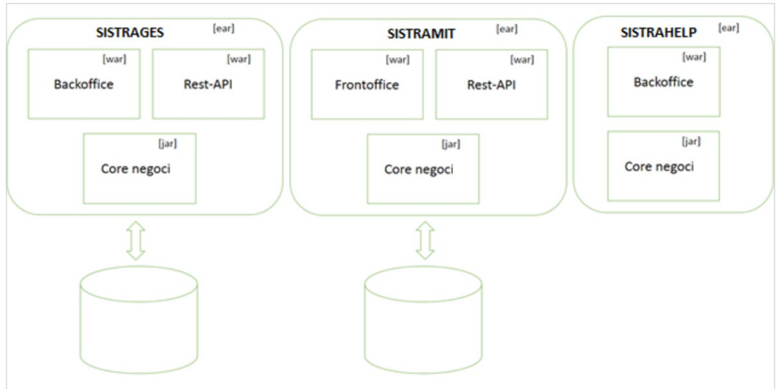
Figura 1: Diagrama dels mòduls de Sistra2
