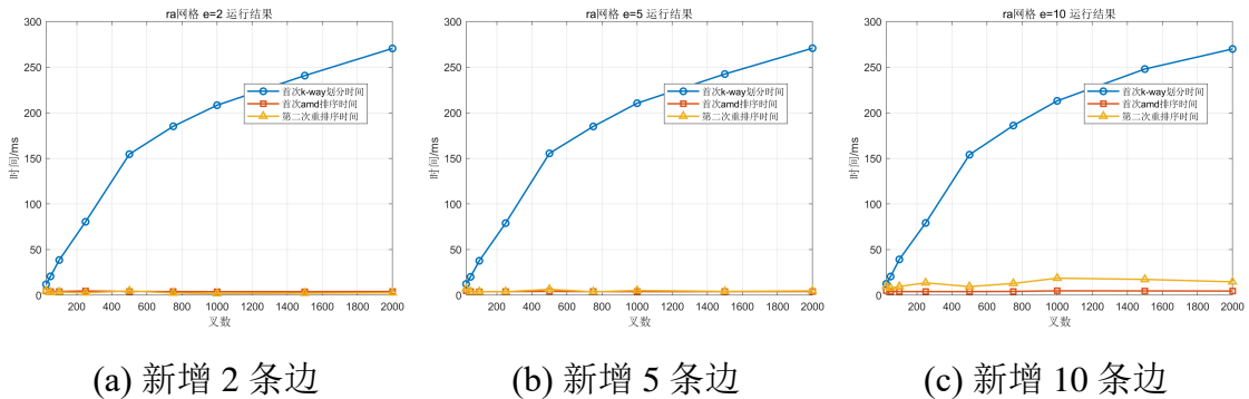
图 4.2 ra 网络运行时间 (ms)
