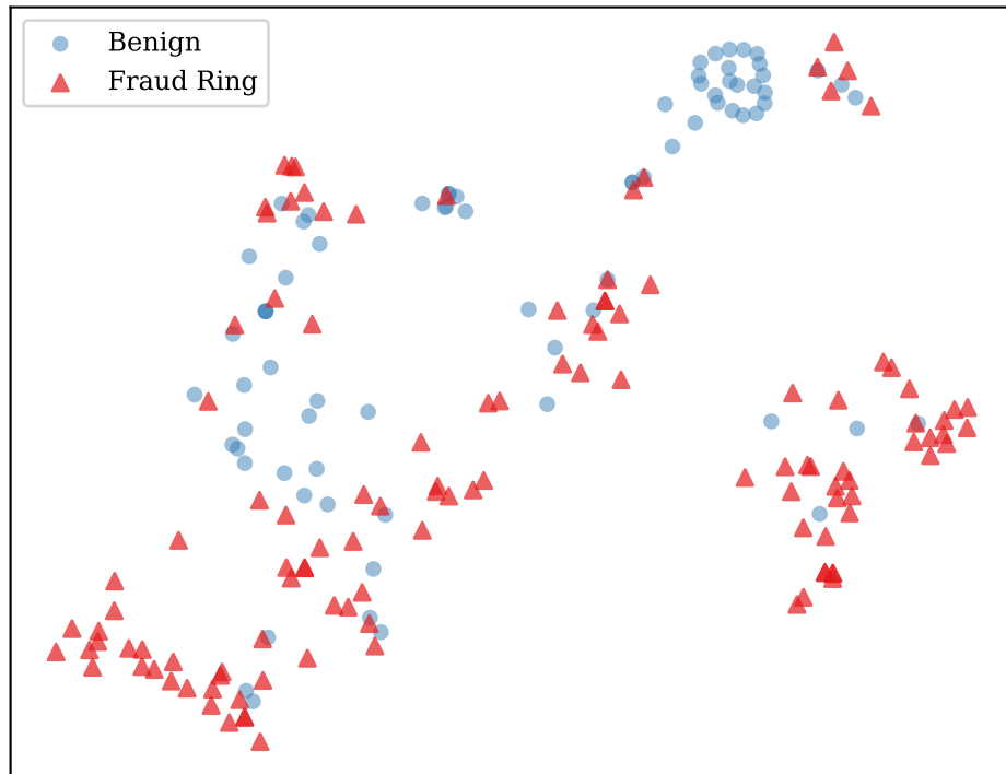
SubGNN+CSP-reg
