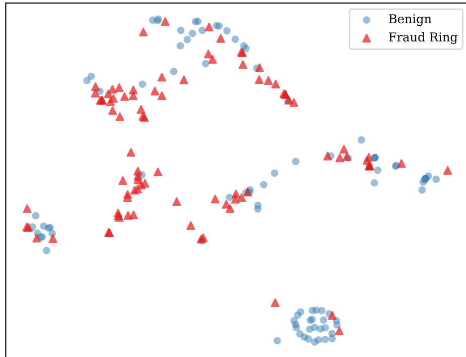
SubGNN+CSP-reg
