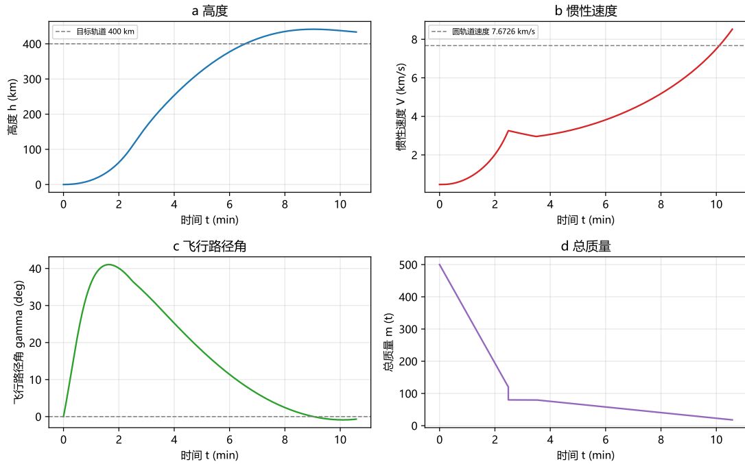
图 4 基准策略全程仿真曲线
