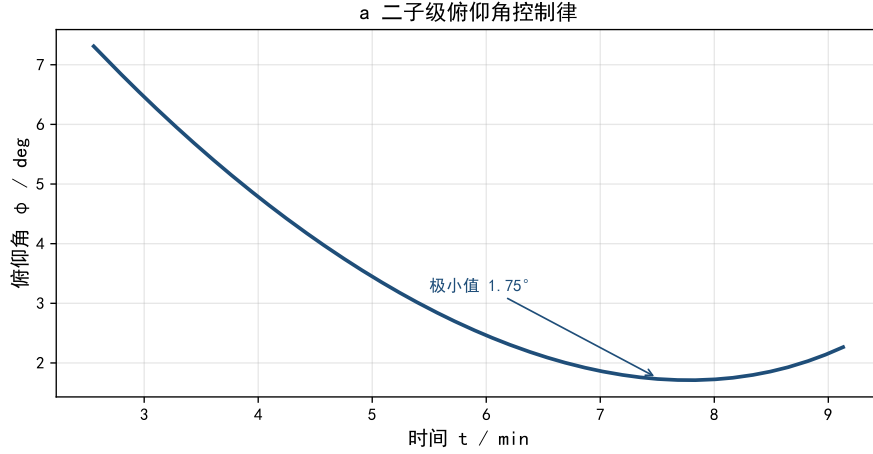
图 8 问题三最优俯仰角控制律
