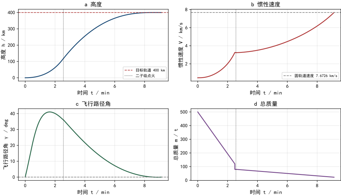
图 7 问题三最优解飞行曲线
