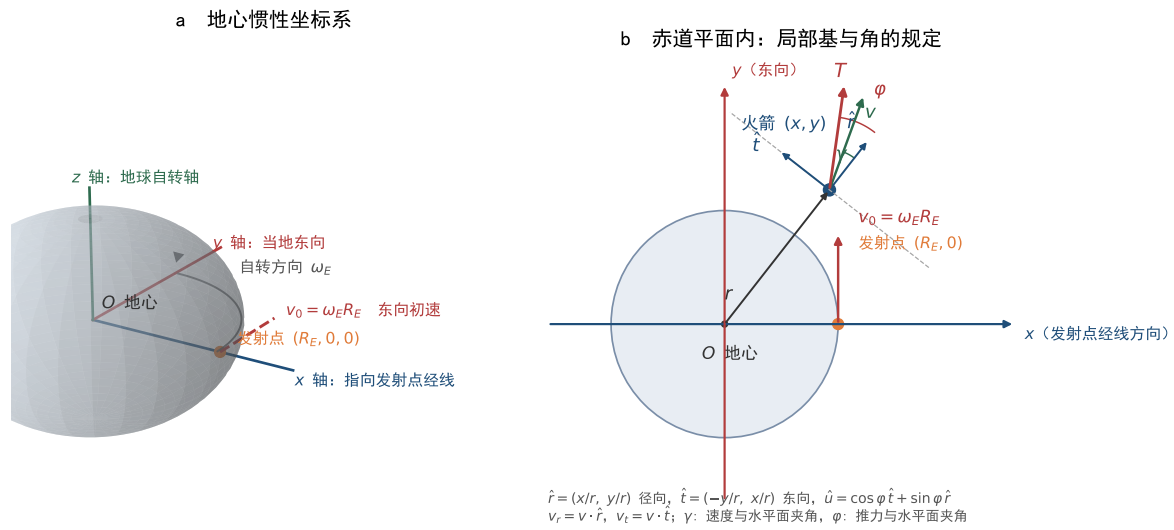
图 1 坐标系与方向规定
