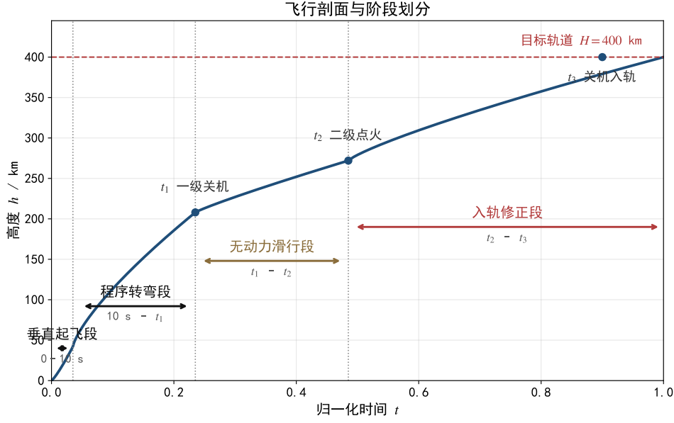
图3 飞行剖面
