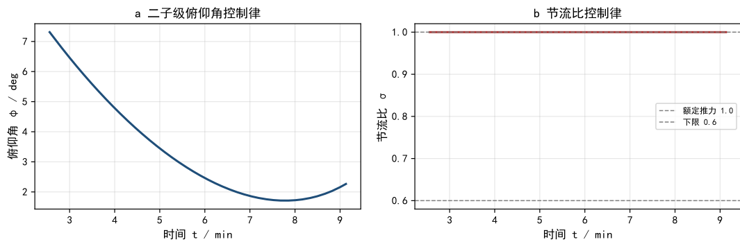
图 10 问题四最优控制律
