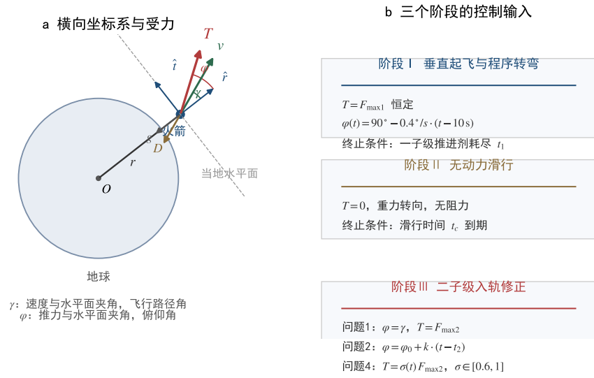
图 1 受力分析
