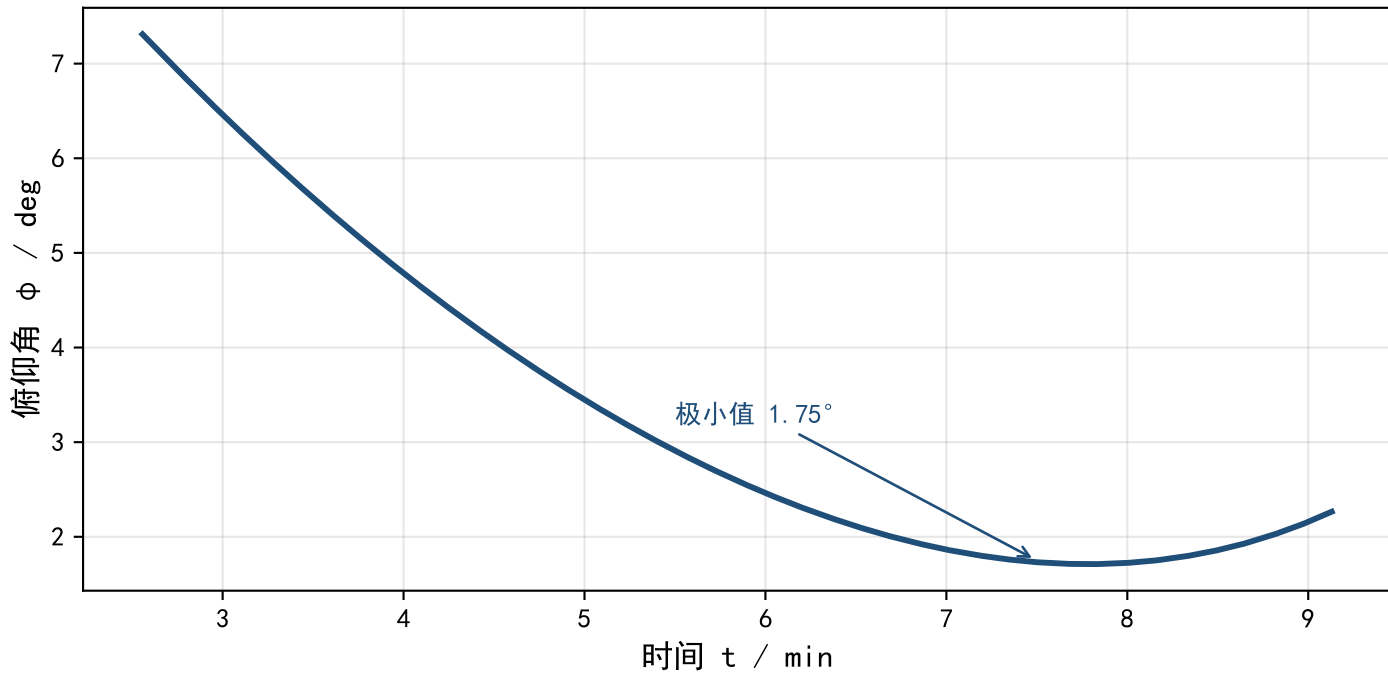
a 二子级俯仰角控制律
