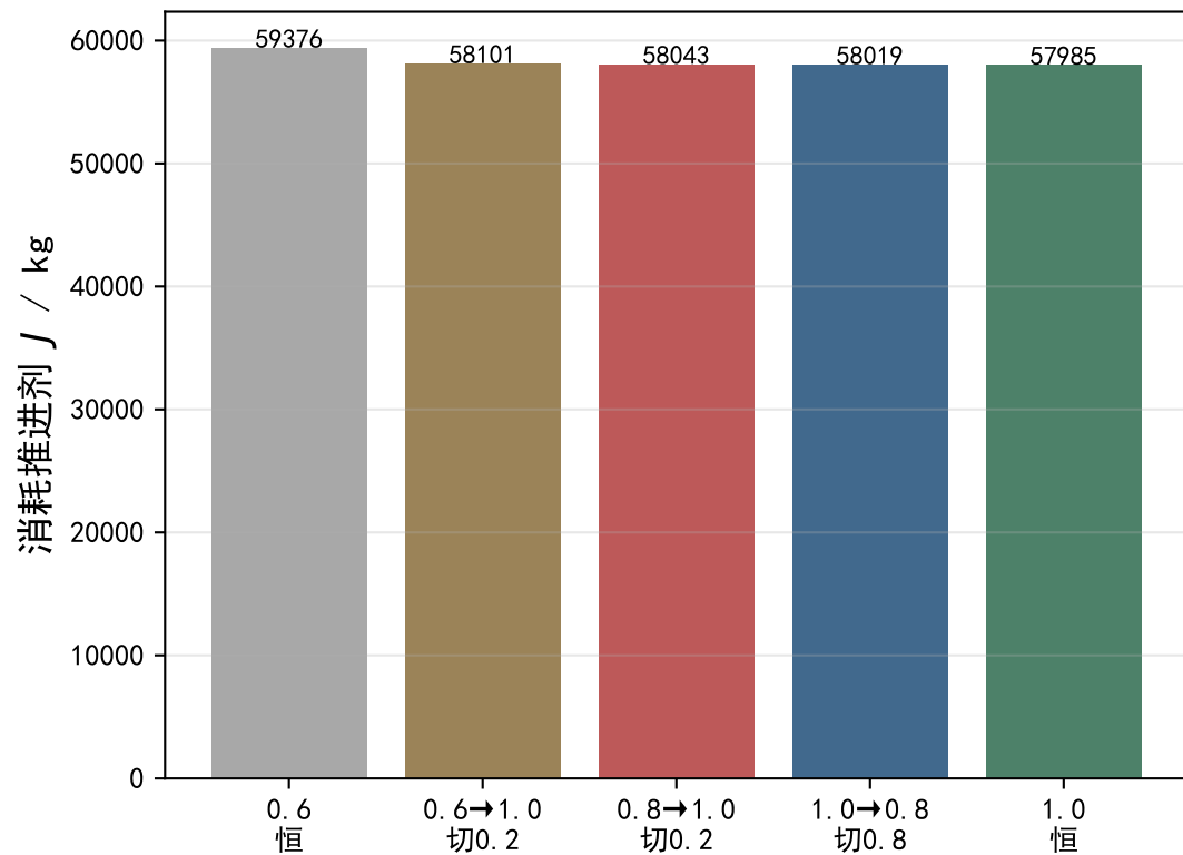
b 两段阶跃节流枚举
