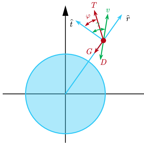
图 2 受力分析
