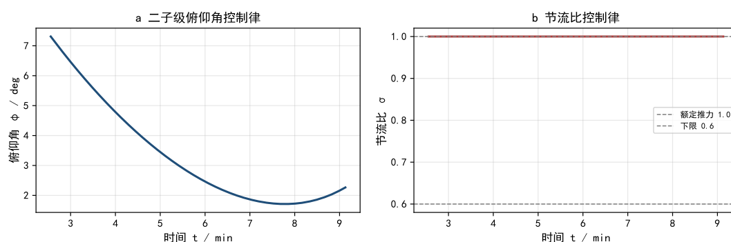
图 10 最优控制律
