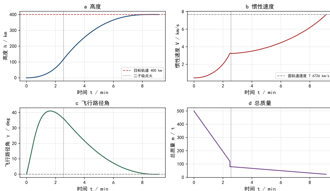
图 9 最优解飞行曲线
