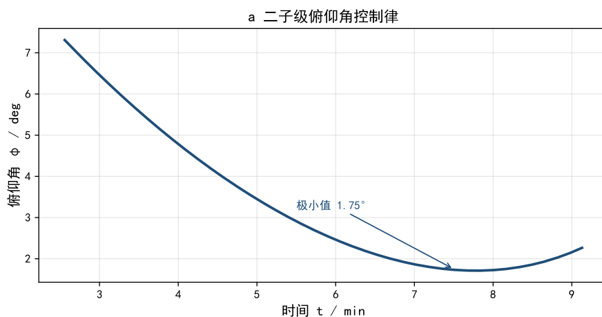
图 8 最优俯仰角控制律
