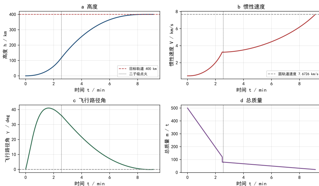
图 7 最优解飞行曲线
