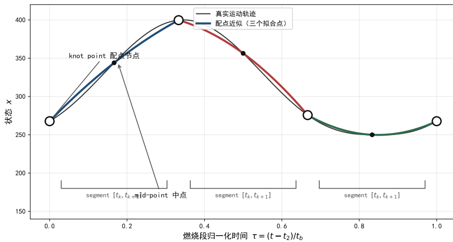
图 6 直接配点法示意
