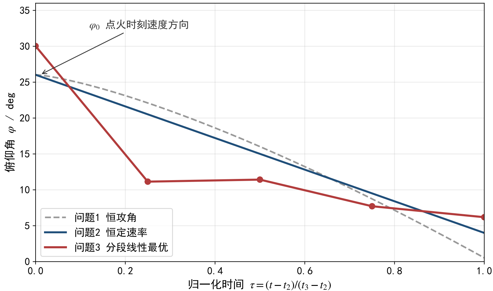
三种控制策略下的俯仰角律
