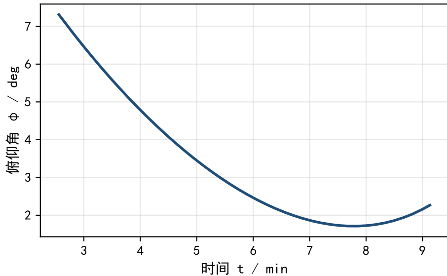
a 二子级俯仰角控制律
