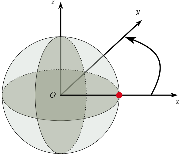
图 1 地心惯性坐标系
