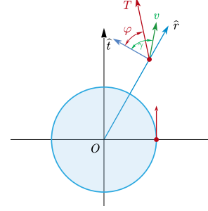
图 2 赤道平面内的局部基与角规定
