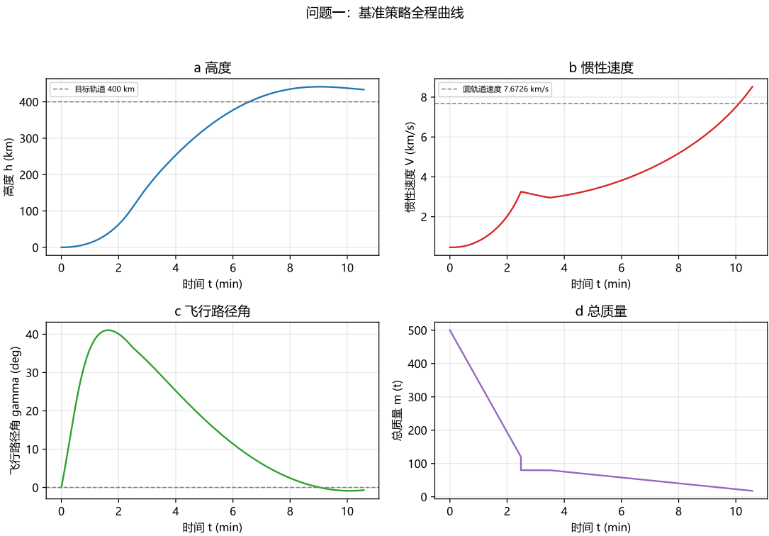
图 5 基准策略全程仿真曲线
