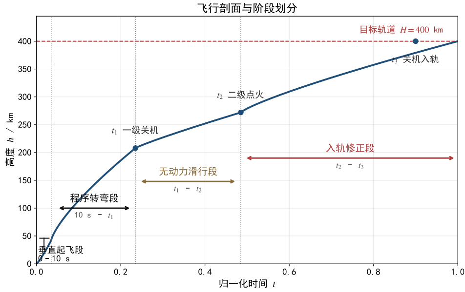
图 4 飞行剖面
