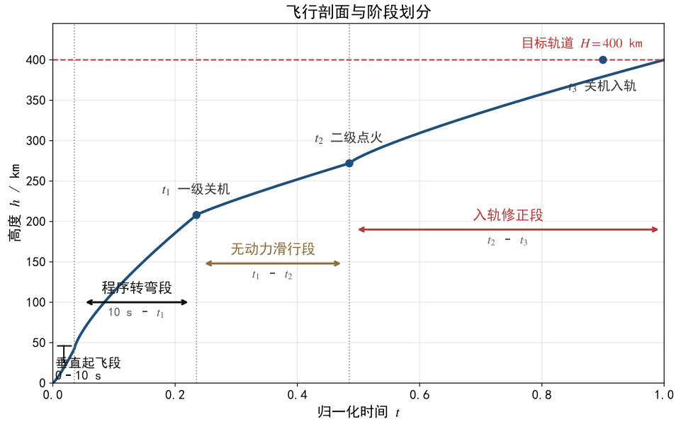
图 4 飞行剖面
