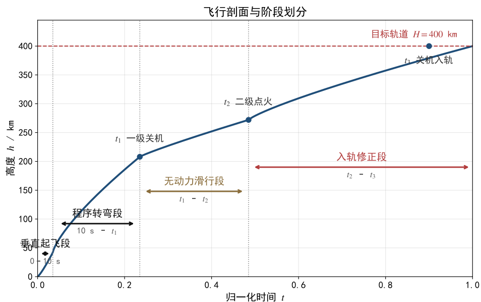
图 2 飞行剖面
