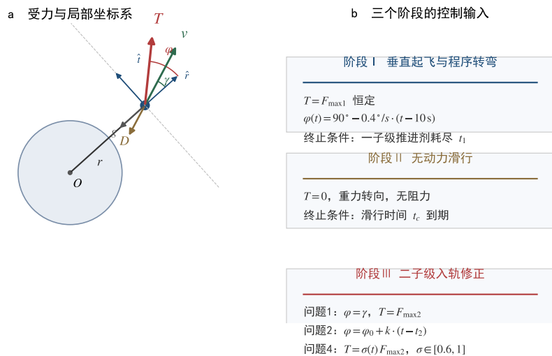
图 1 受力分析
