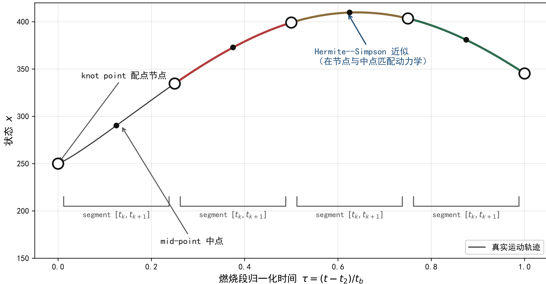
直接配点法：节点、中点与分段上的动力学匹配
