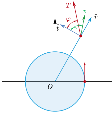
图 2 赤道平面内的局部基与角规定
