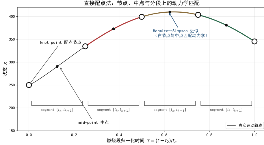
图 7 直接配点法示意
