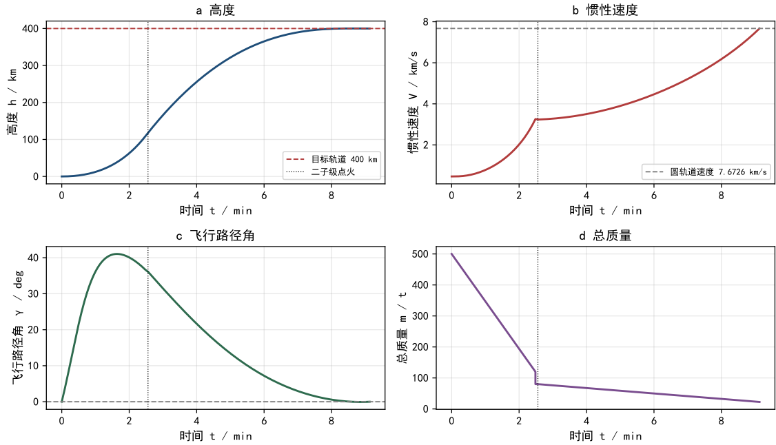
图 8 最优解飞行曲线
