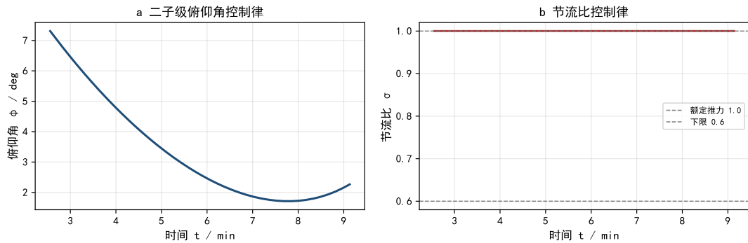
图 11 最优控制律
