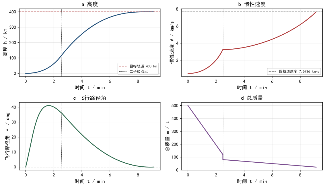
图 10 最优解飞行曲线
