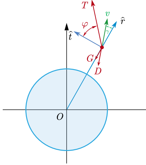
图3 受力分析
