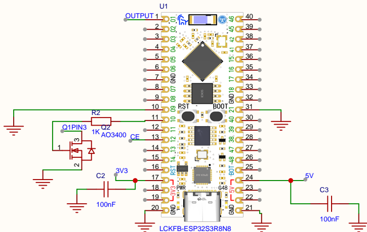
单片机模块
