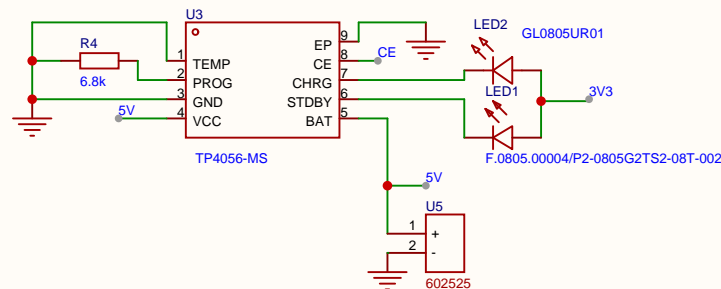
电源模块
