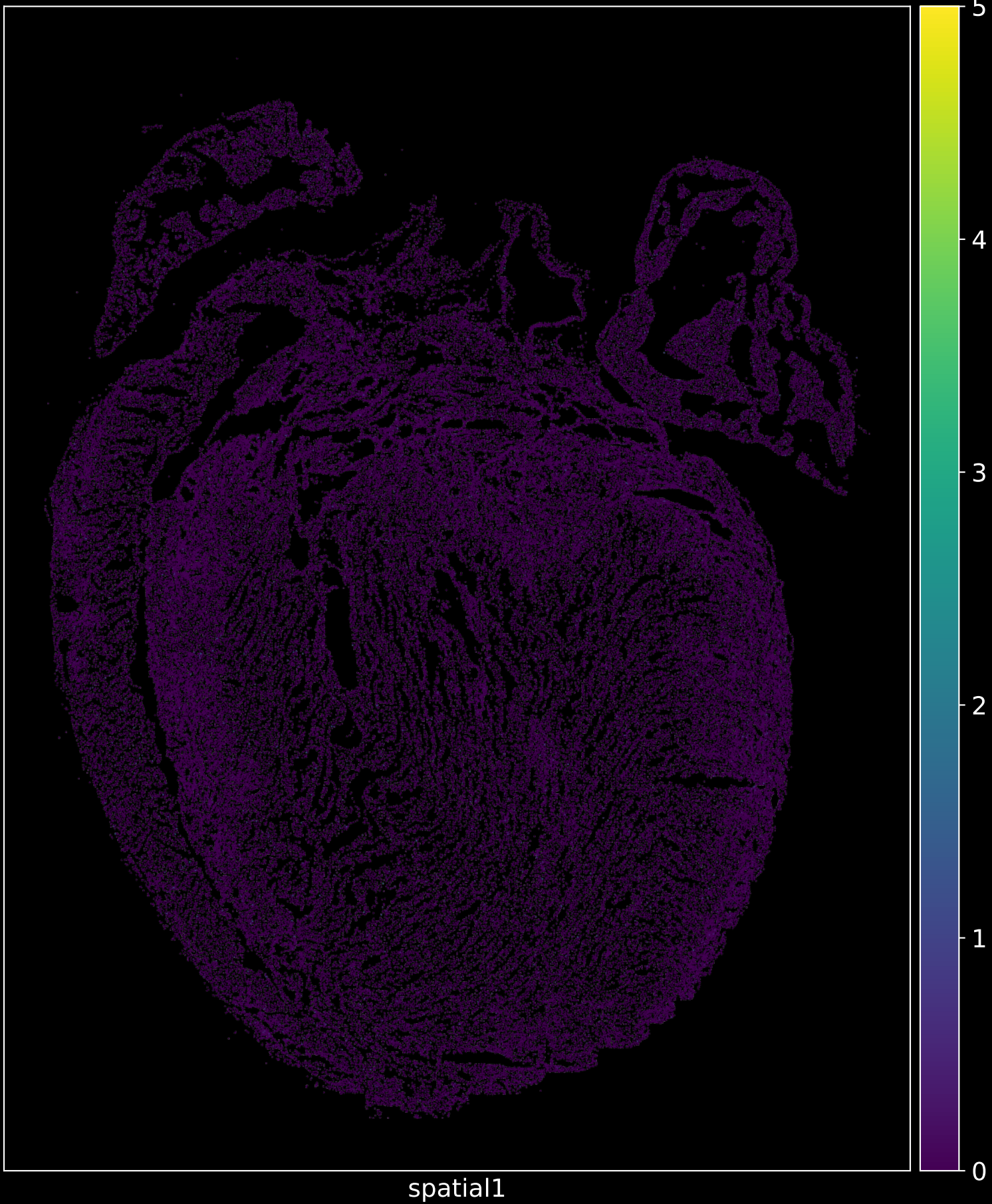
Smad4 in KO1
