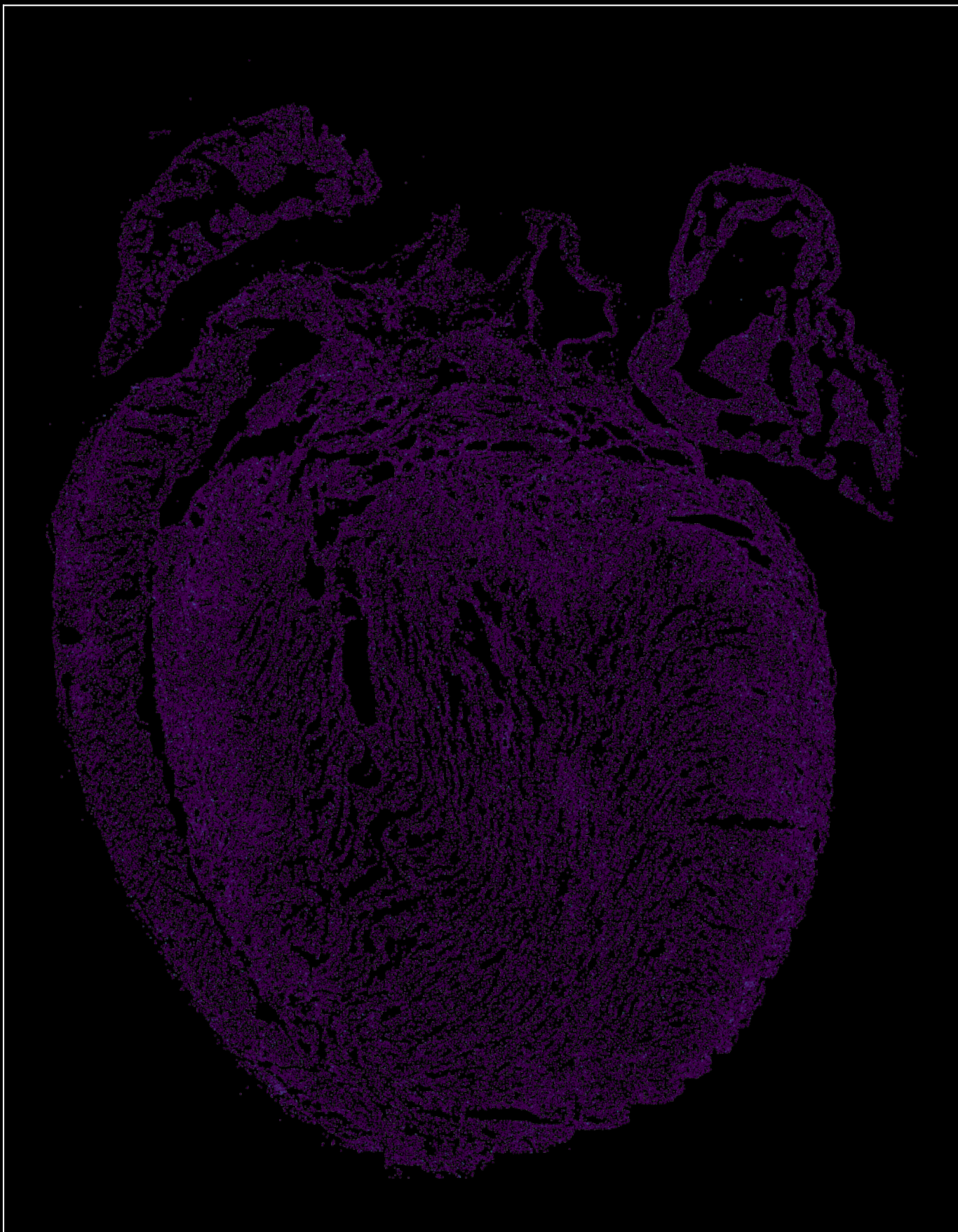
Arhgap15 in KO1
