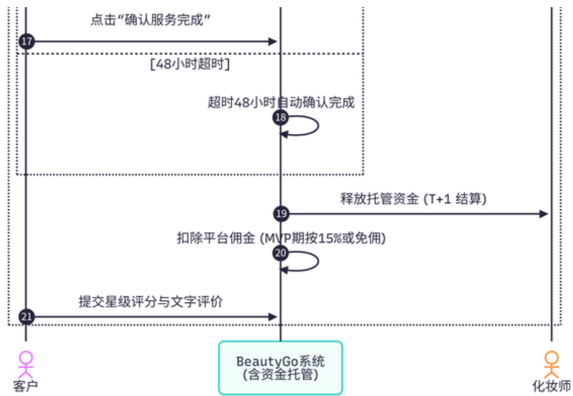
MVP 核心流程时序图
