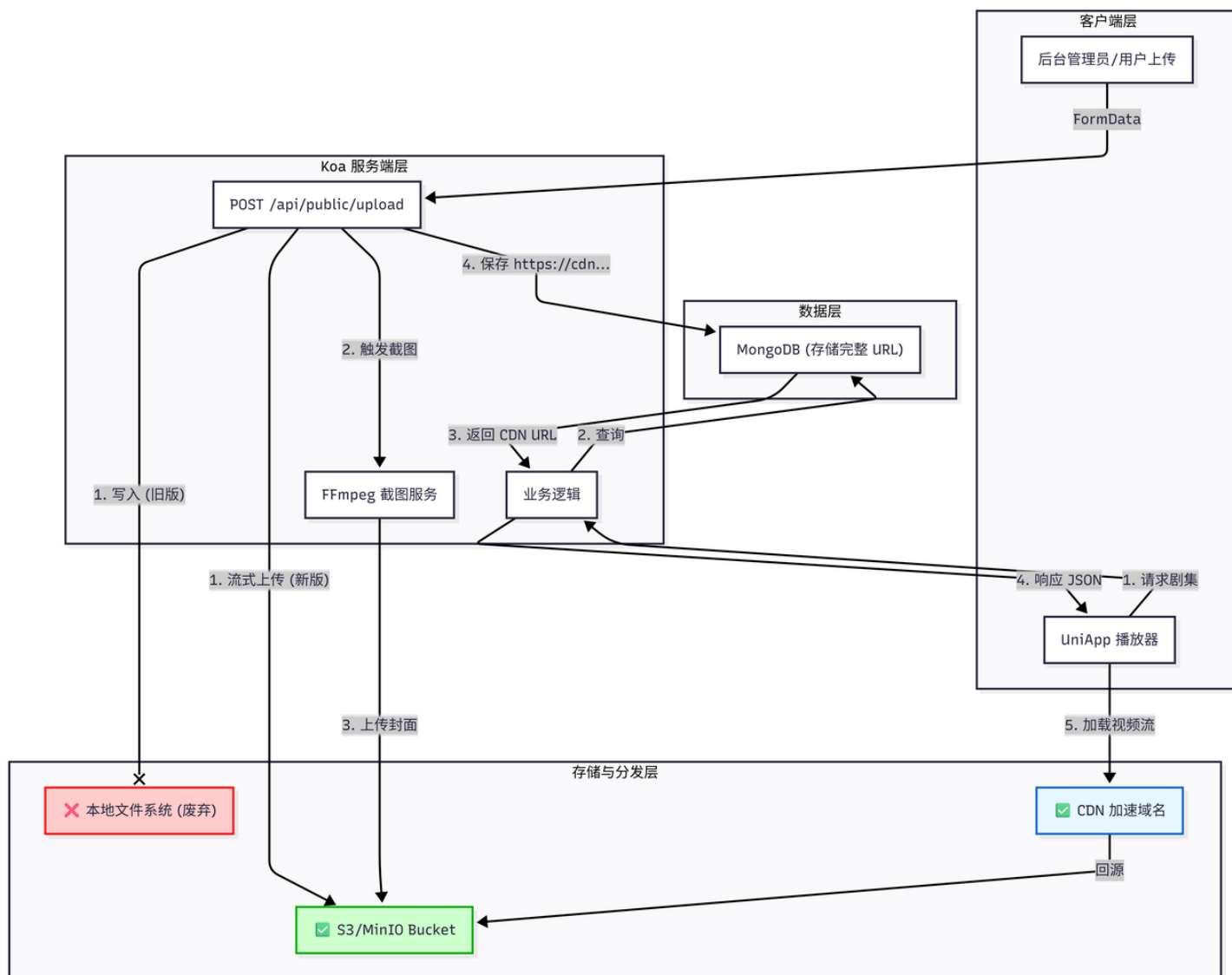
存储架构改造数据流图
