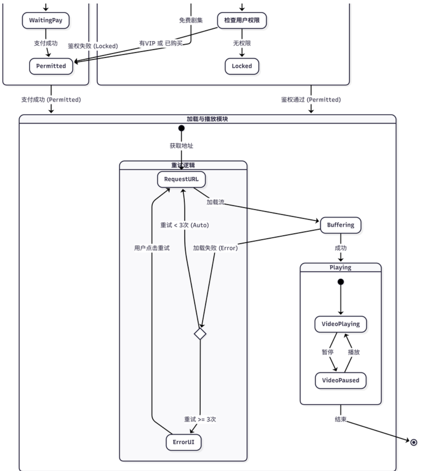
播放器容错与鉴权状态机
