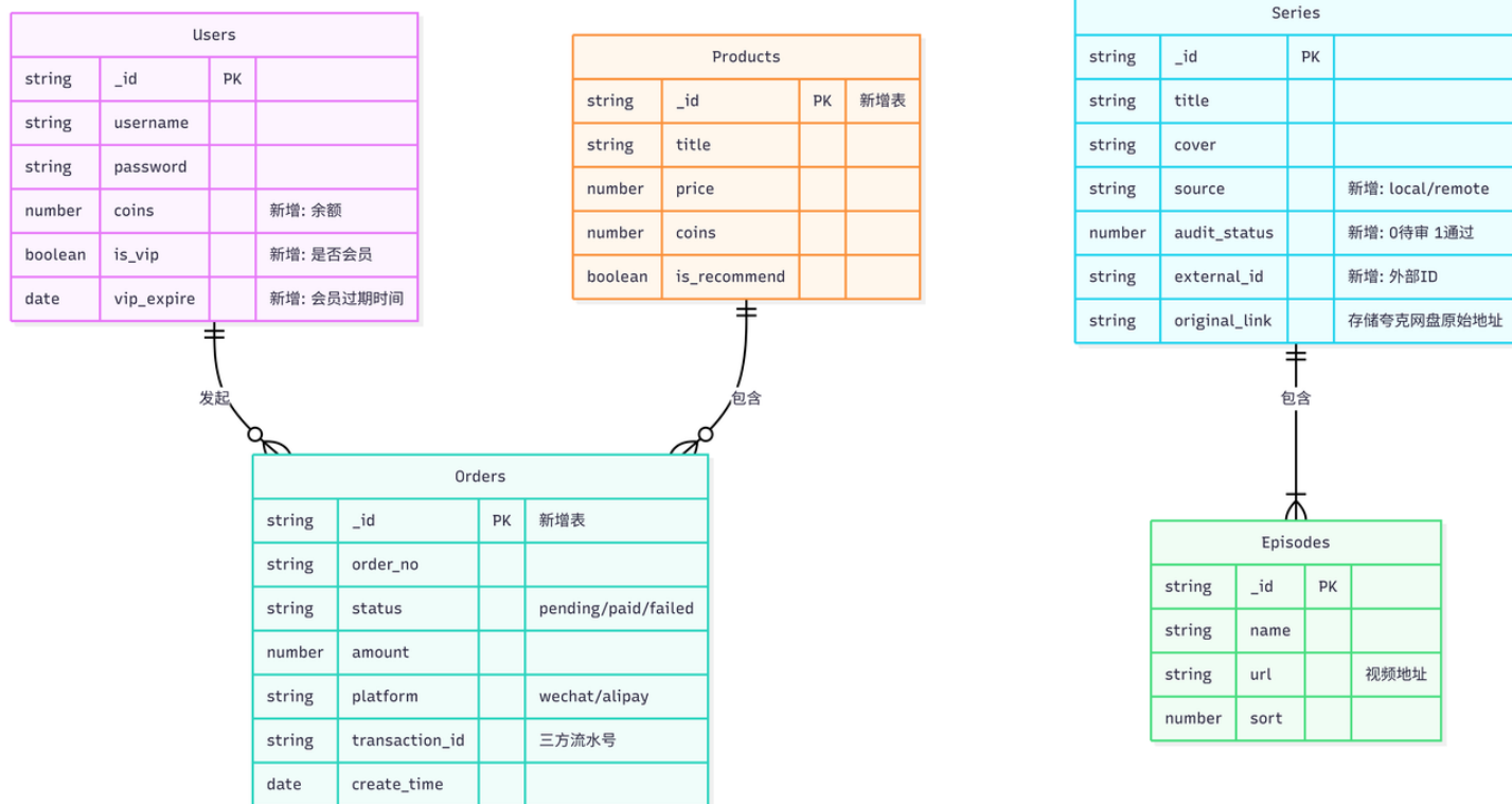
数据库实体关系图
