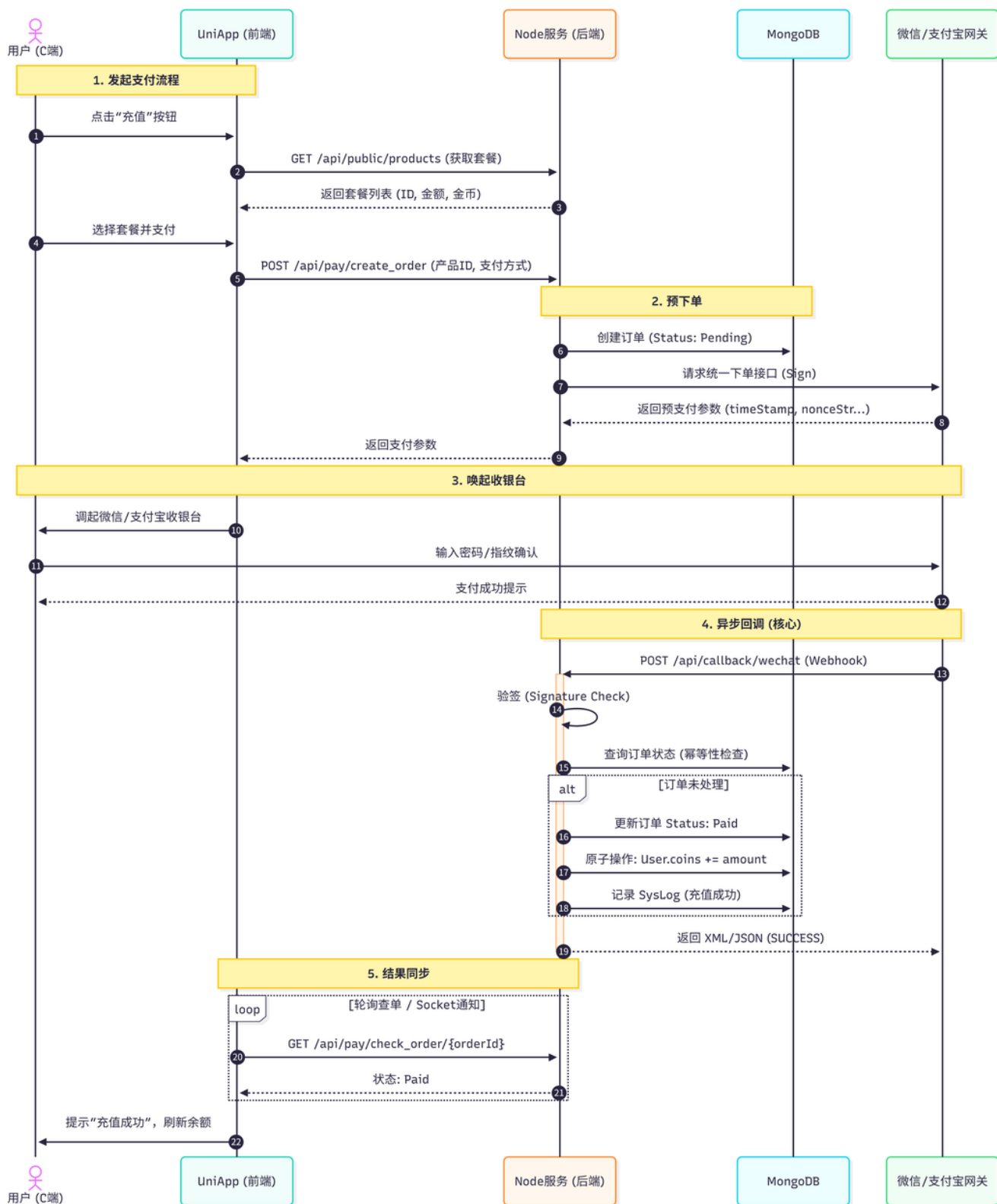
支付业务时序图
