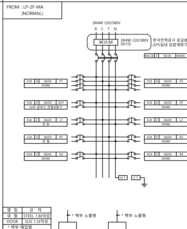
LP-2F-A1, A2, A3, A4(근생1, 2, 3, 4)
