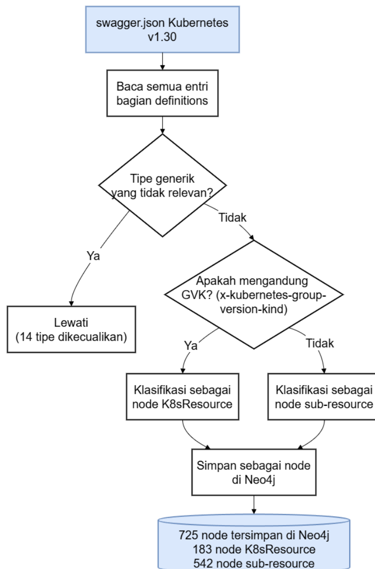
Gambar V.1 Alur fase 1: Pembuatan Node Definition dari swagger.json
