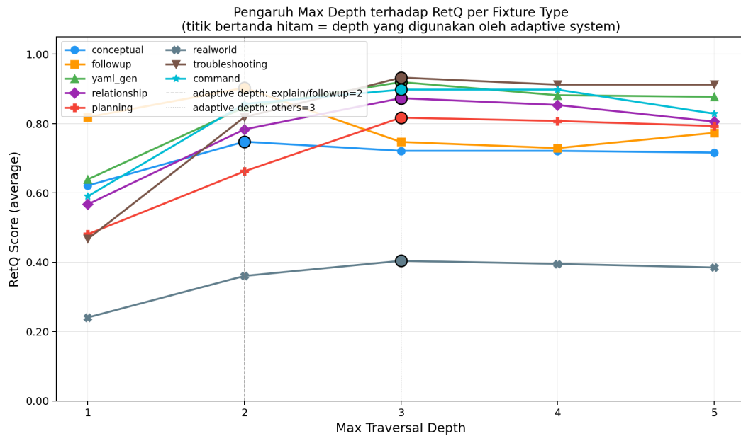
Gambar V.8 Pengaruh kedalaman traversal terhadap RetQ per kategori fixture
