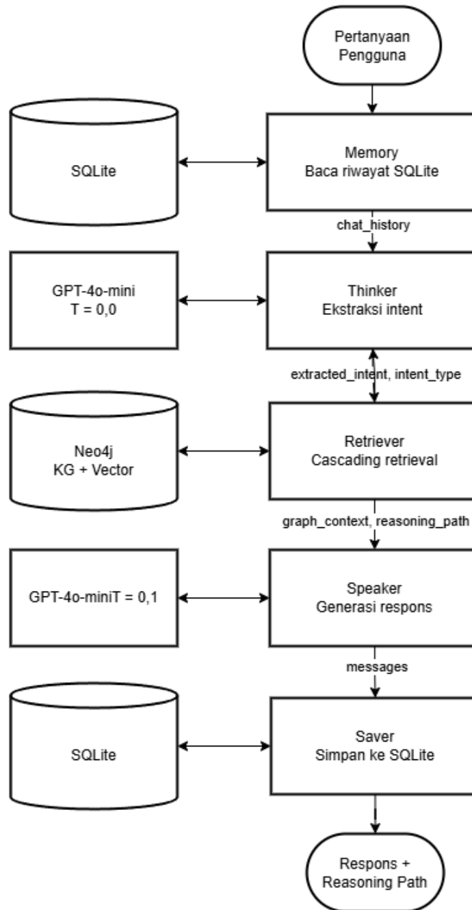
Gambar V.6 Diagram interaksi lima modul agent LangGraph
