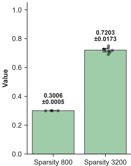
FVU
