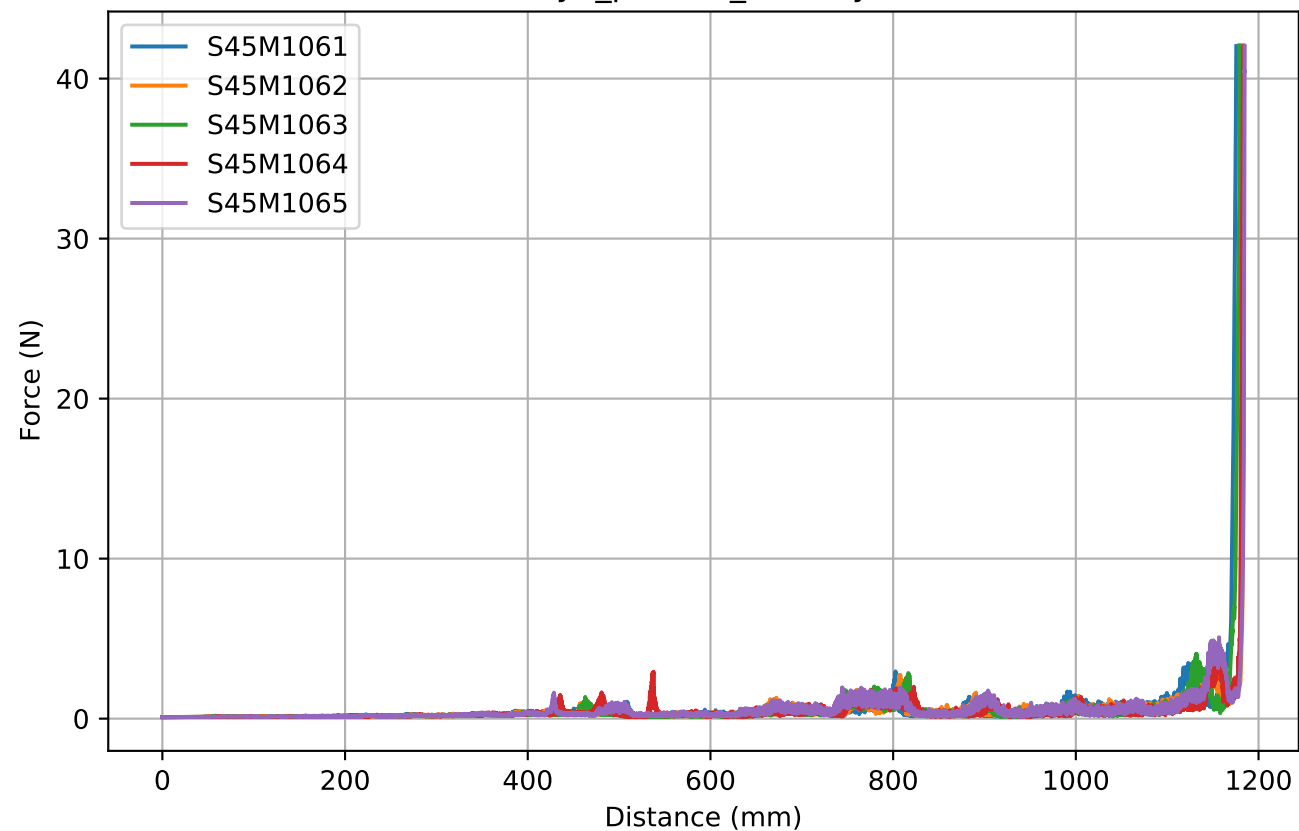
day1_profiles_velocity8
