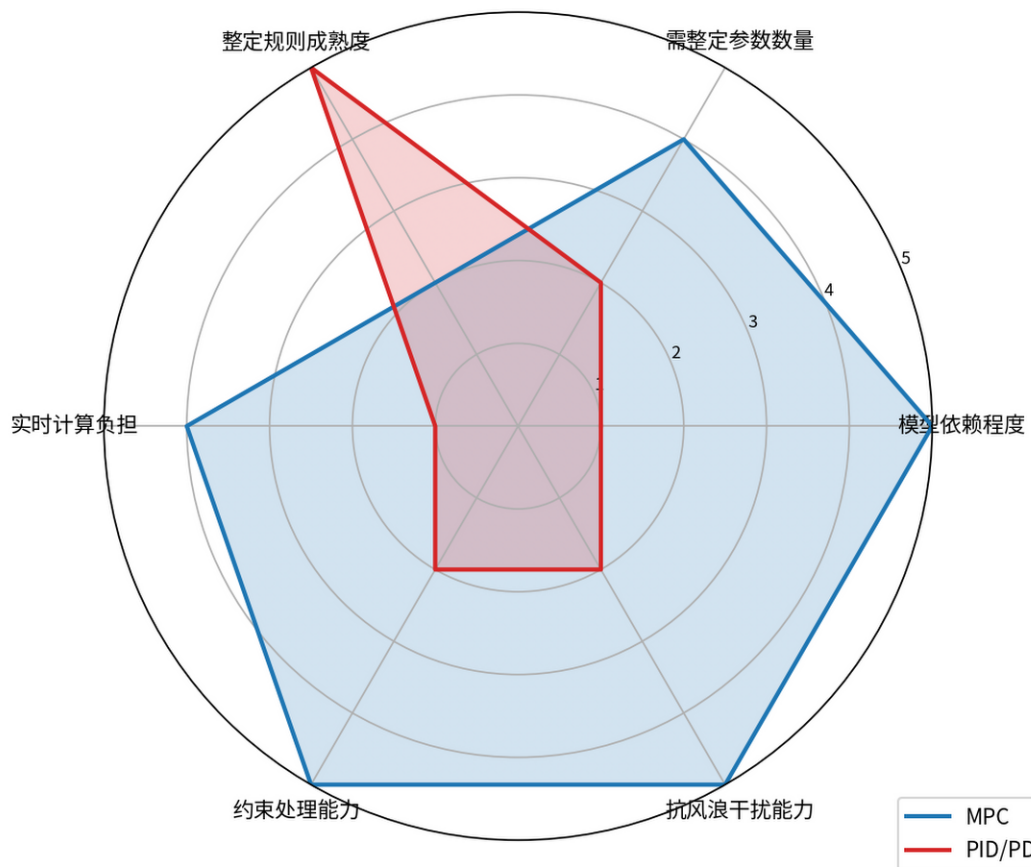
图3 MPC vs PID/PD 工程特性雷达图 (1-5 分) 前四项为负担维度 (越大越难)，后两项为能力维度 (越大越好)
