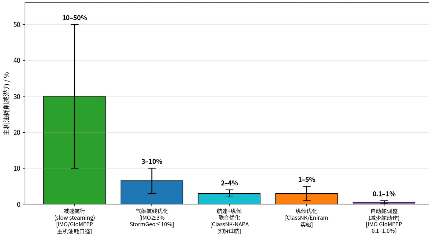
图4 船舶节能措施的节油量级对比（区间上下限，来源：IMO / 船级社 / 实船试航）
