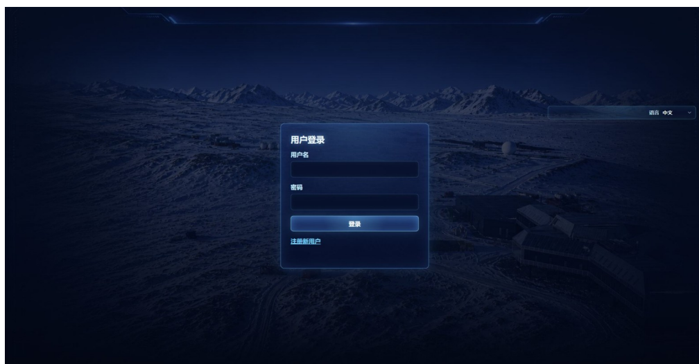
图4 登录页面
