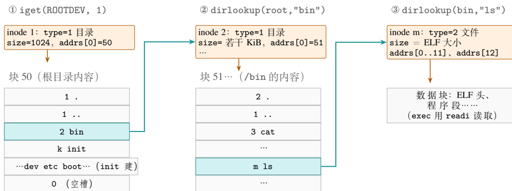
图 6.8: namei("/bin/ls") 的查找过程。目录本身也是文件，内容是一串目录项； namex() 每次用 skipelem() 取出一个路径分量，在当前目录的内容里 dirlookup() ，得到下一个 inode。块号 50、51 是 mkfs 的分配顺序决定的，k、m 取决于 Makefile 里程序的排列顺序
