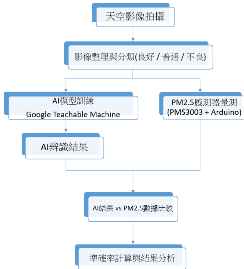
▲ 圖三：實驗架構流程圖（第二作者繪製）
