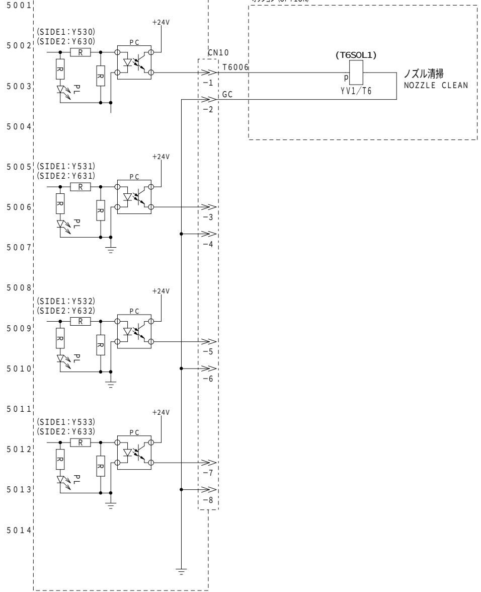
デバイスパレットI/O基板 (T1PCB2) DEVICE_PALETTE_I/O_PCB
