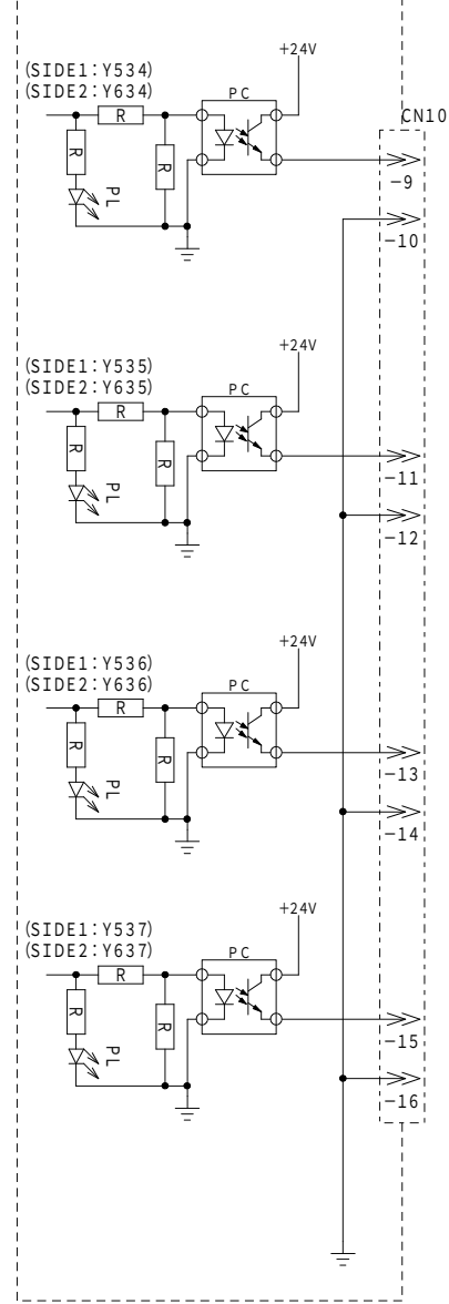
デバイスパレットI/O基板 (T1PCB2) DEVICE_PALETTE_I/O_PCB
