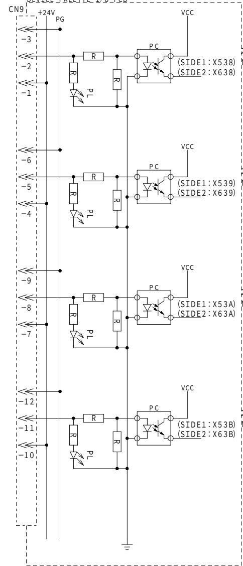
デバイスパレット I/O 基板 (T1PCB2) DEVICE_PALETTE_I/O_PCB
