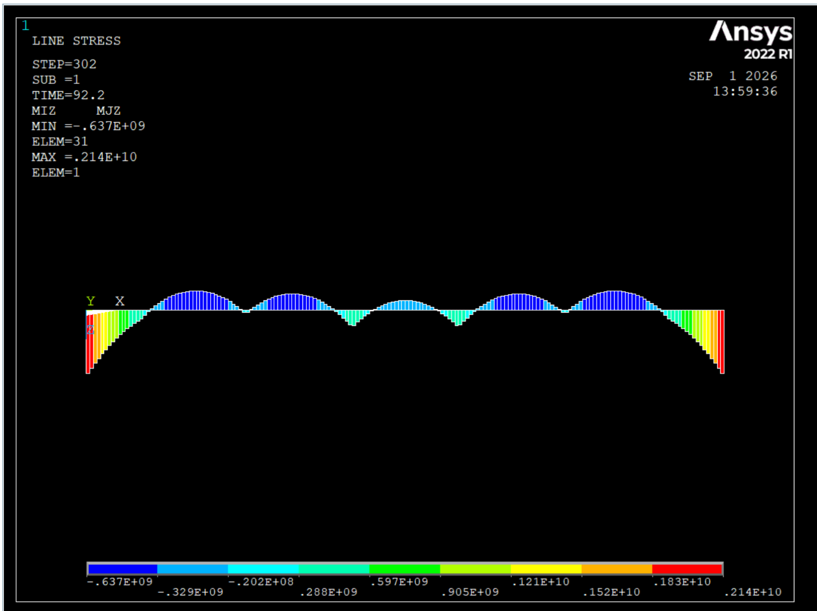
图3 管体弯矩图 (Y方向视图)
