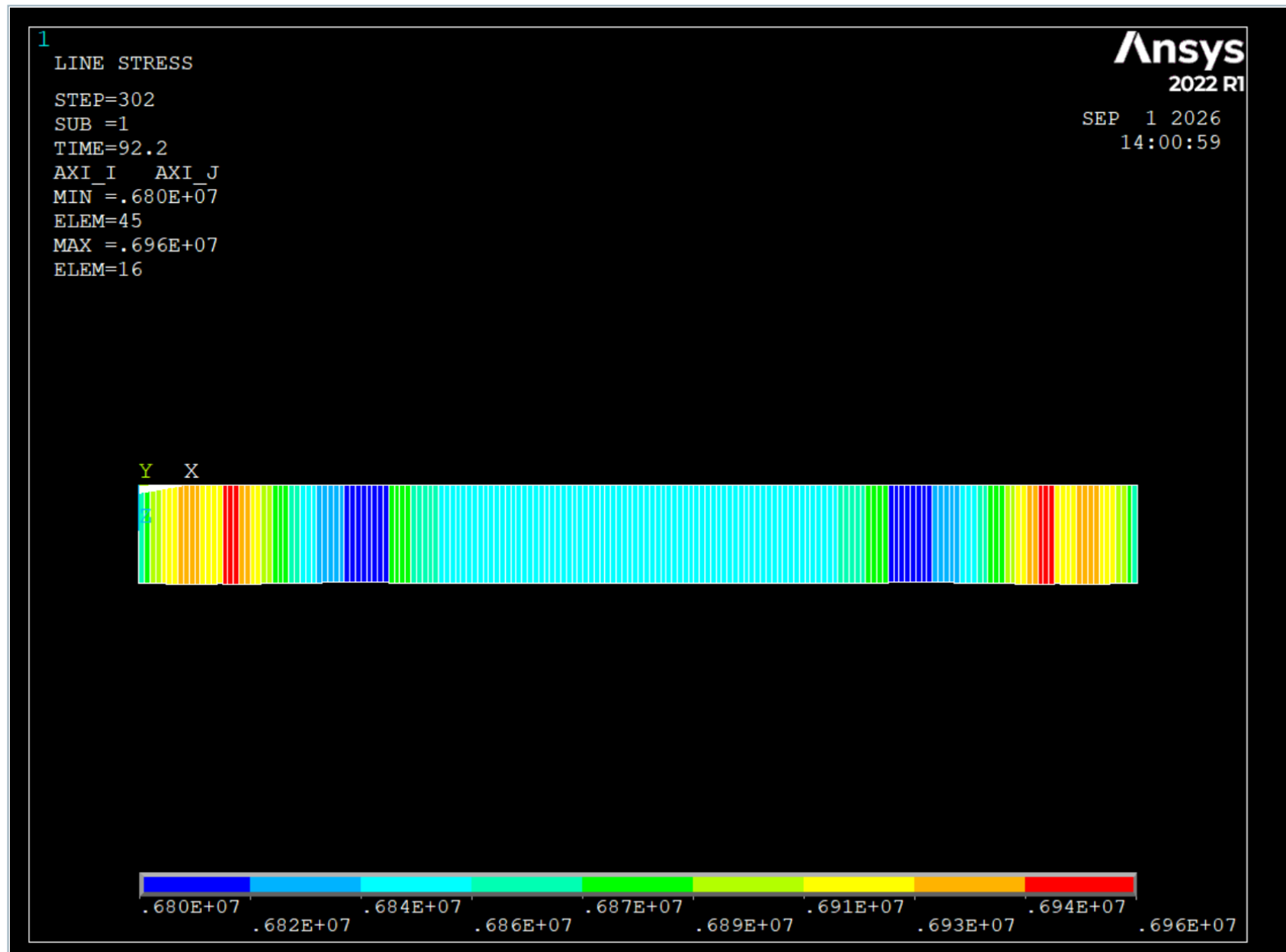
图8 管体轴力图 (Z方向视图)
