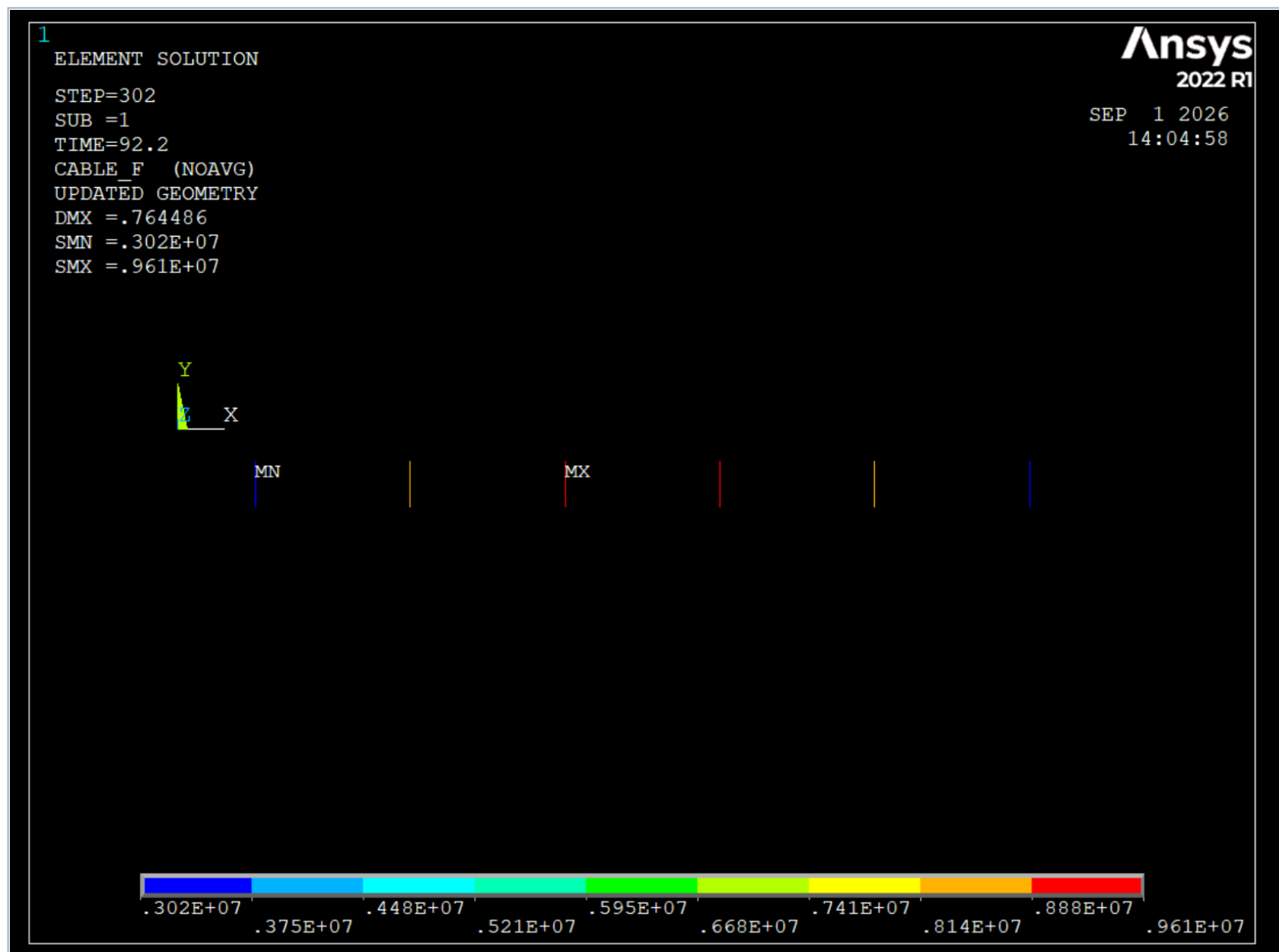
图10 竖向锚索轴力分布图
