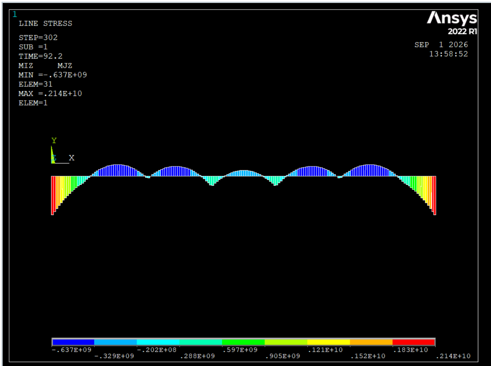
图2 管体弯矩图 (Z方向视图)
