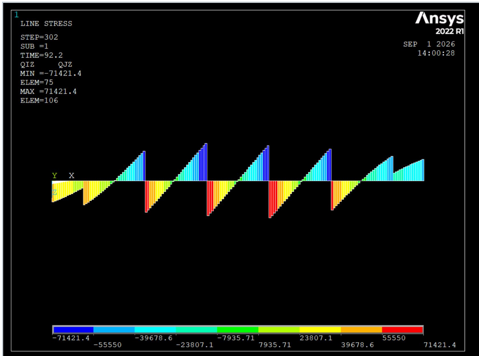
图4 管体剪力图 (Z方向视图)
