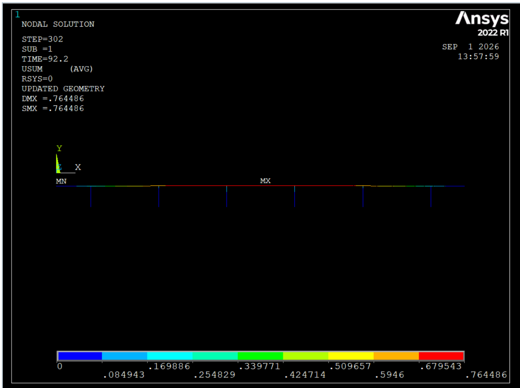
图1 管体总位移云图 (USUM)
