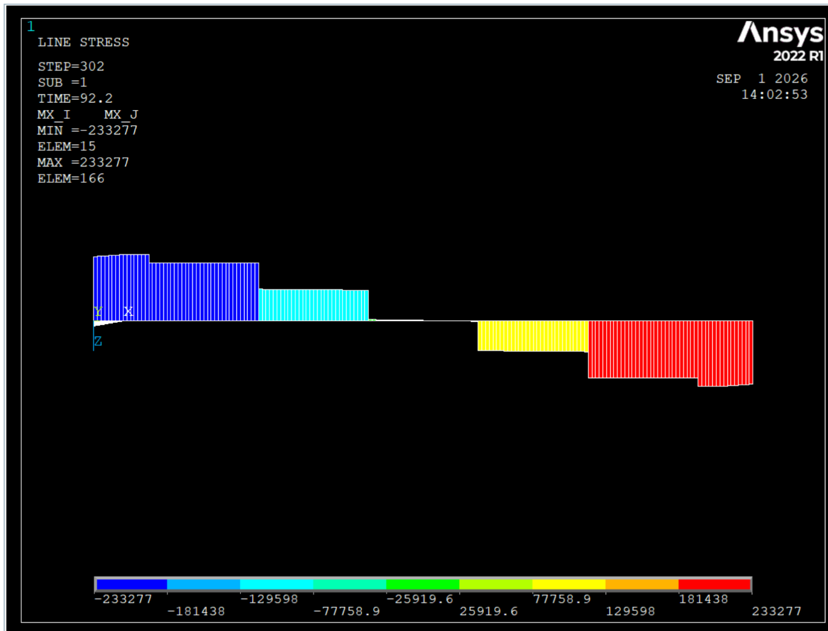
图7 管体扭矩图 (Y方向视图)
