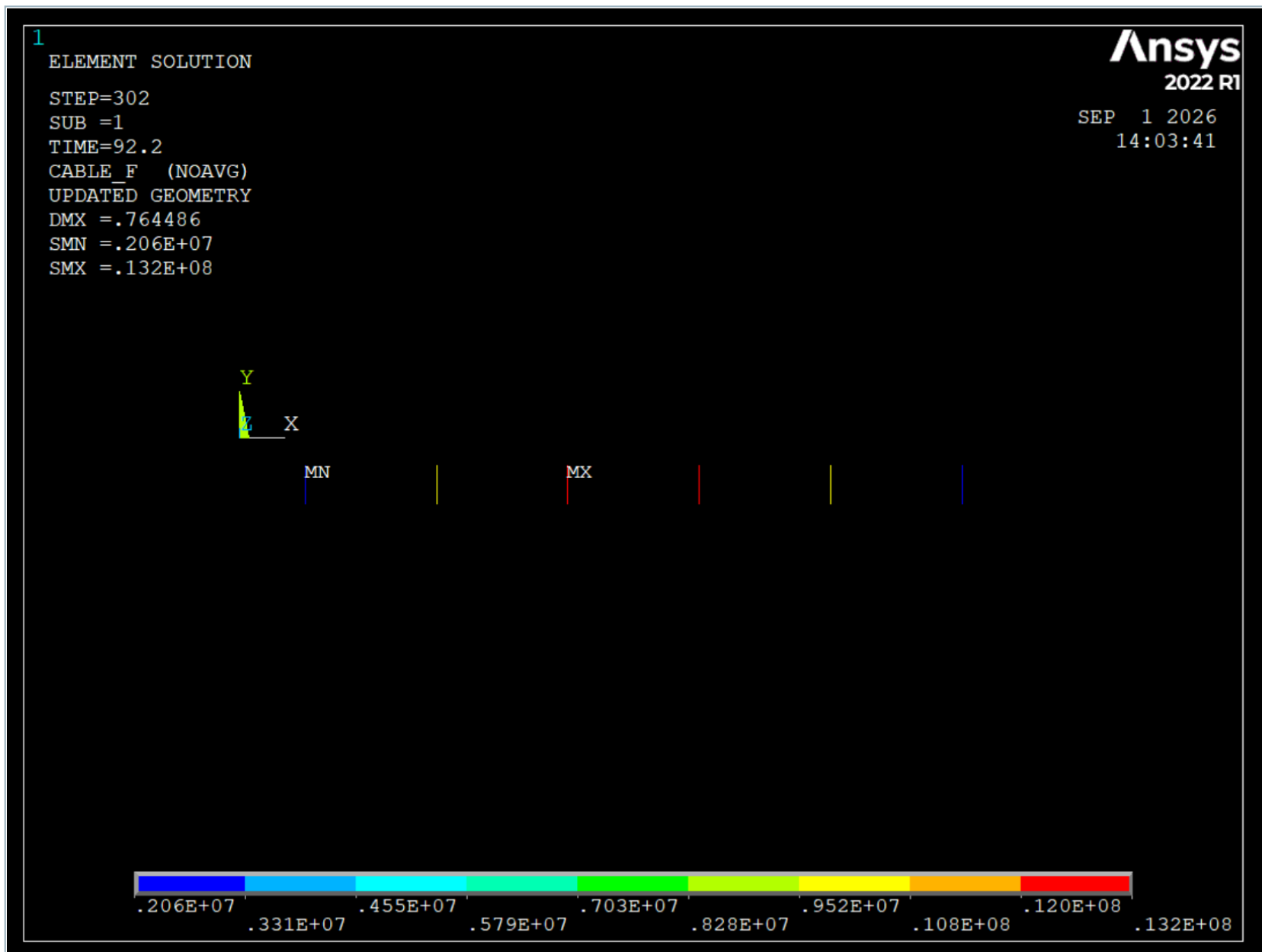
图11 斜向锚索轴力分布图
