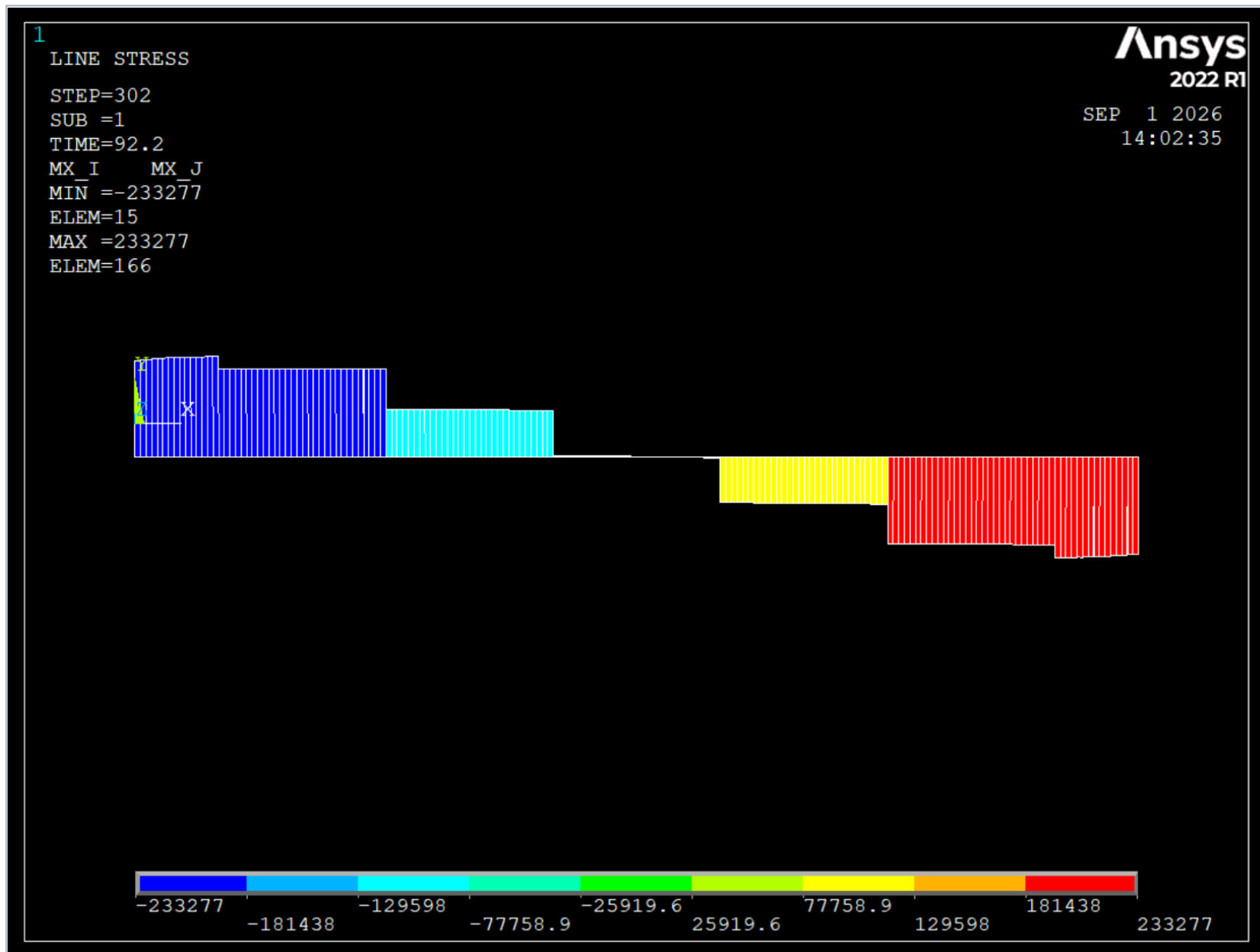
图6 管体扭矩图 (Z方向视图)
