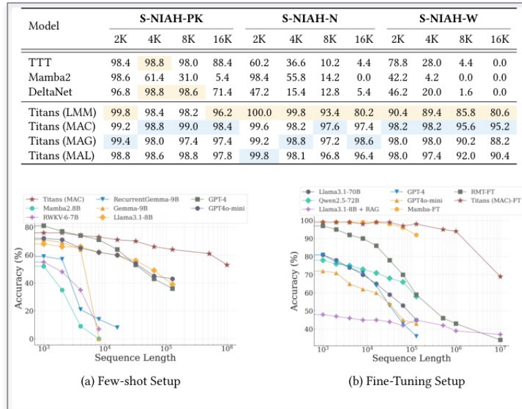
Figure 6 — BABILong: MAC 가 GPT-4 · Mamba 2.8B · RWKV 7B 를 앞섬 ( 적은 파라미터로 )
