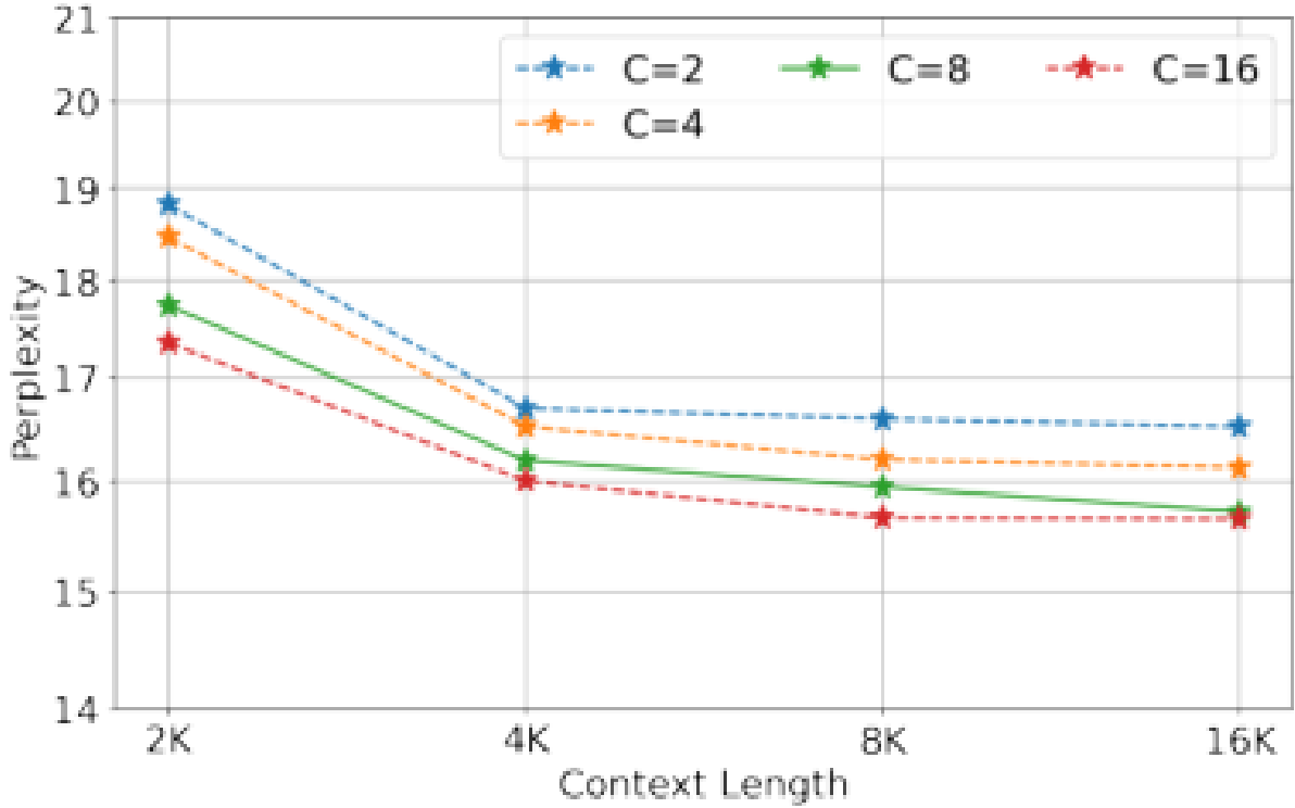
그림 5: OmegaNet 에서 국소 문맥 길이 c 가 서로 다른 전역 문맥길이별 성능에 주는 효과. 출처: 원저자, arXiv:2505.23735 Fig.5
