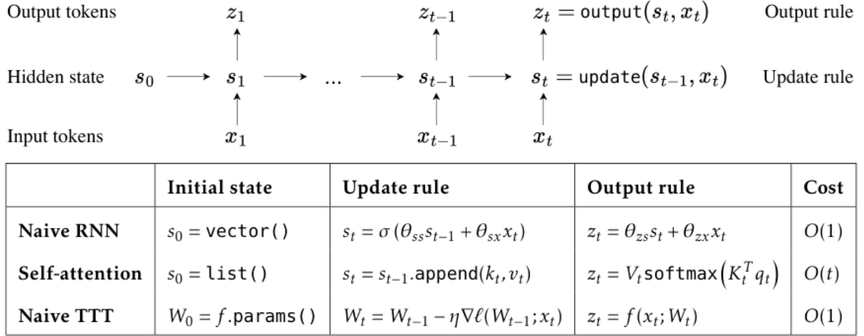
그림 8-1 — 모든 sequence modeling layer 를 “hidden state + update rule” 의 한 틀로 보고, naive RNN·self-attention·naive TTT 를 세 요소 (initial state, update rule, output rule) 의 서로 다른 instantiation 으로 나란히세운 그림. TTT 의 update rule 은 self-supervised loss \ell 에 대한 gradient step 이고, 상태가 고정 크기라 read cost 가 O(1) 이다. 출처: Sun et al. 2024, Learning to (Learn at Test Time) (arXiv:2407.04620), 원문 Fig. 3 —원저자의 그림 (third-party), 본서의 결과가 아님.
