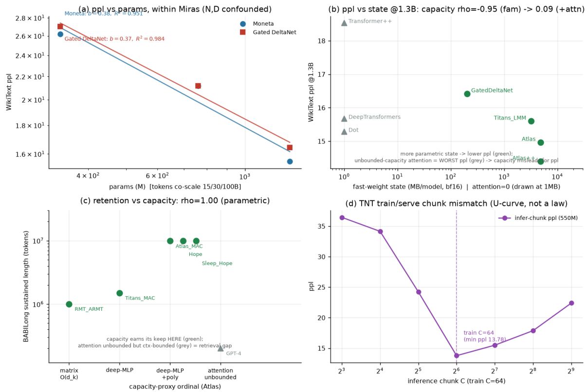
그림 25-1: 여섯 편 (params, tokens, ppl/score) 점을 digitize 해 맞춘 candidate scaling fit; exploration-grade 의 ordering 만 load-bearing.
