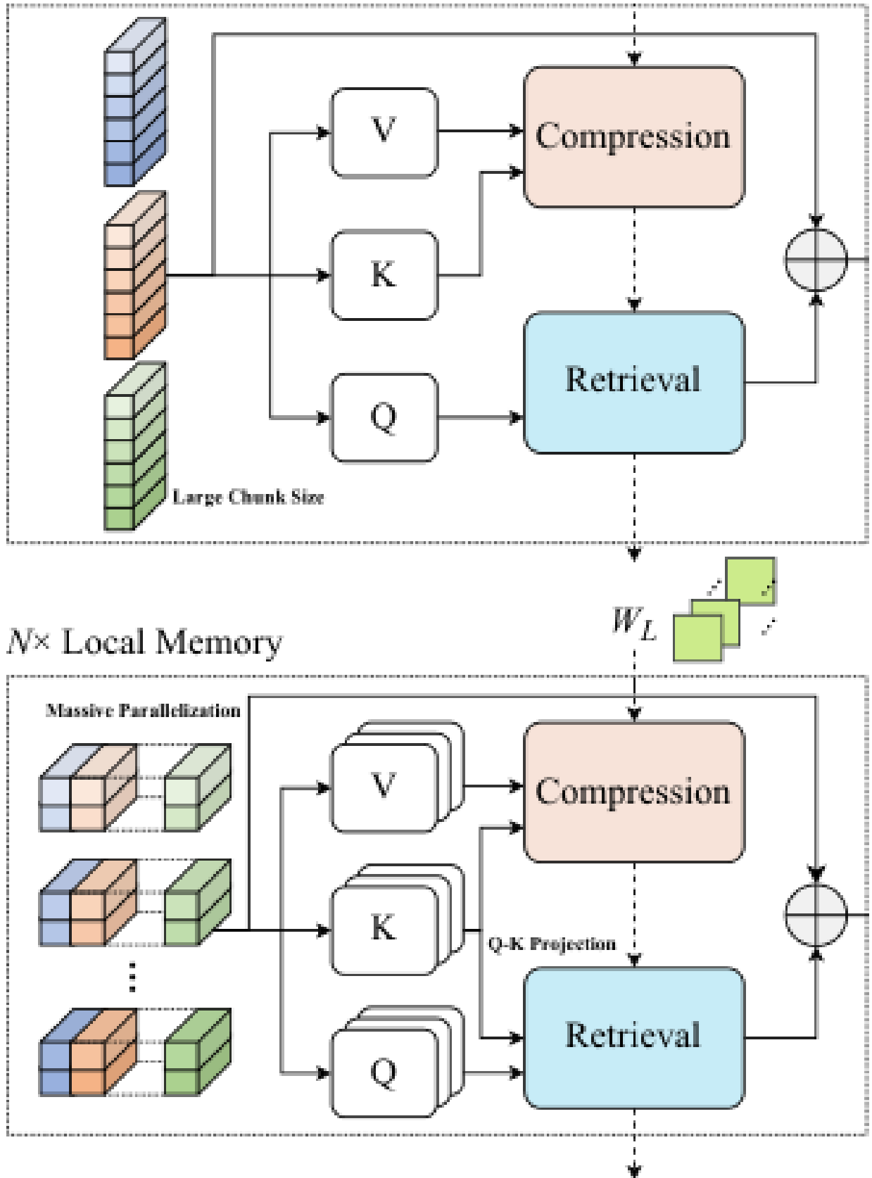
TNT Stage 1 의 아키텍처 개관. 위 블록: 큰 chunk 로 순차적으로도는 하나의 global memory(long-range 담당). 아래 블록: 학습된 초기상태에서 주기적으로 재초기화되어 대량 병렬화(Massive Parallelization) 되는 N 개의 local memory. 두 메모리 모두 Compression(write)·Retrieval(read) 두 연산을 갖고, 두 경로 출력이합산되어 y_t 가 된다 — 단 Q-K Projection 은 local 경로에만 붙는다. 출처: 저자, TNT(arXiv:2511.07343) Fig.3 — 원저자 그림.
