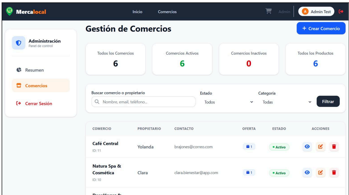
Imagen 26: Área de gestión para el administrador de la plataforma.
