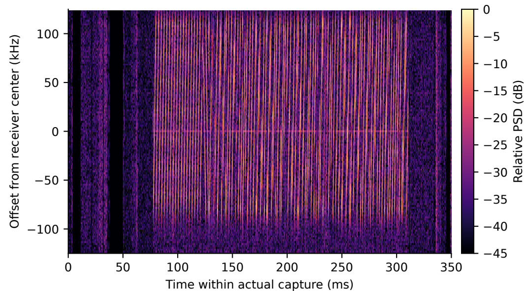
D Real SF9 packet · CRC 3777
