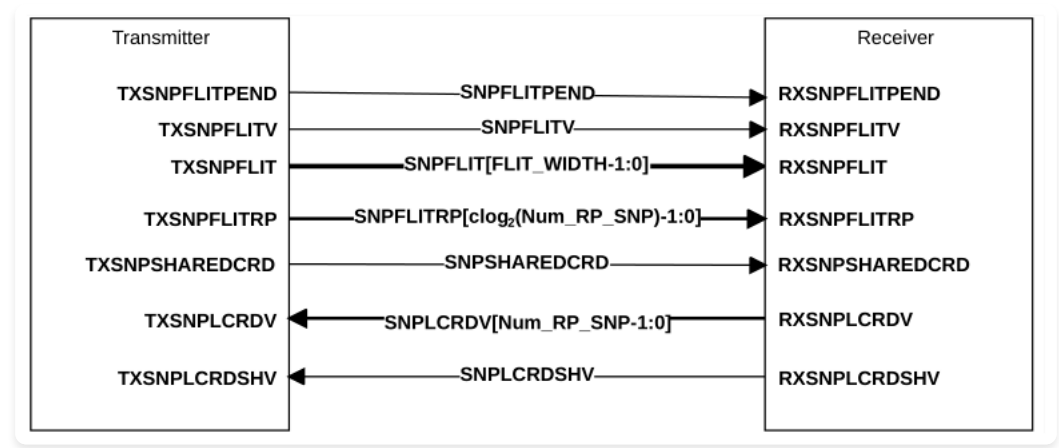
Figure p468 图 B13.13: SNP 通道接口引脚
