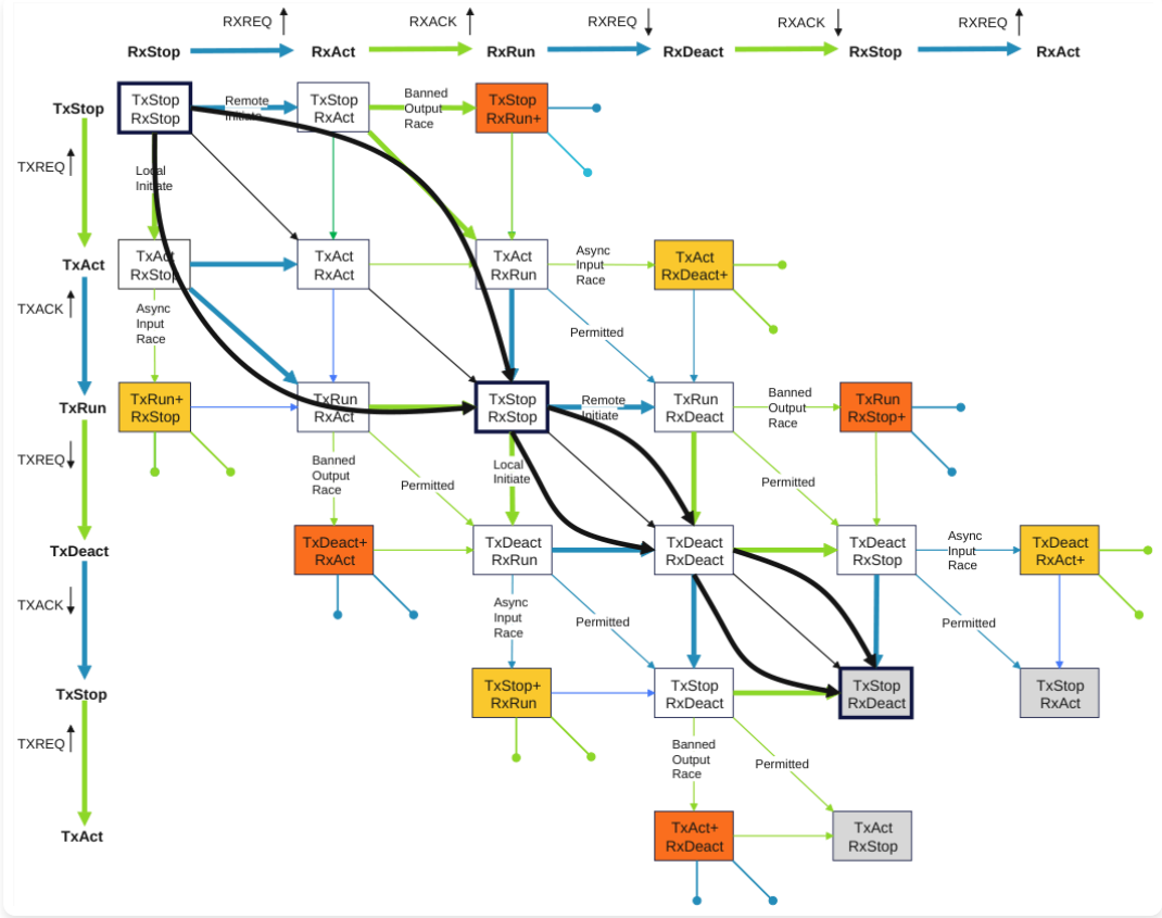
图 p533 图 B14.8：预期的 Tx 与 Rx 状态机转换
