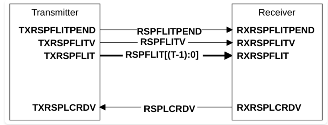
Figure p467 图 B13.12: RSP 通道接口引脚
