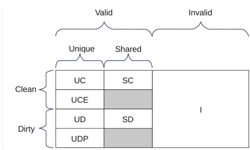
图 B1.3: 缓存状态模型
