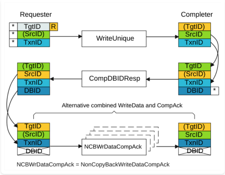
图 B2.31: 使用合并的 WriteData 和 CompAck 响应时的 ID 值传输
