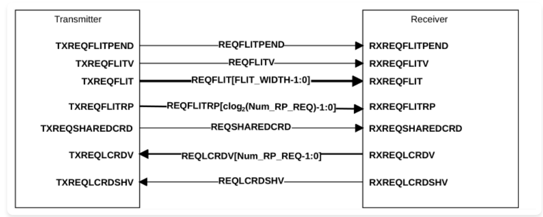
Figure p466 图 B13.11: REQ 通道接口引脚
