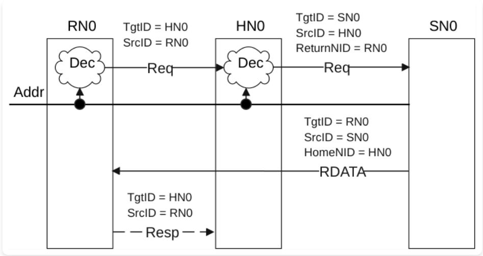
Figure p188 图 B3.1：不进行重映射时的 TgtID 分配
