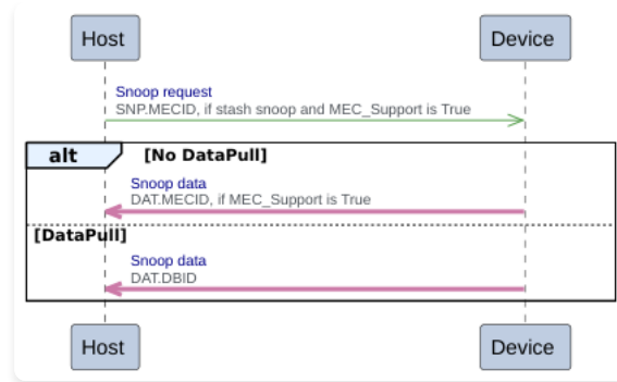
图 B10.5: 主机对已缓存 HCM 位置进行侦听时的 RME-CDA 字段
