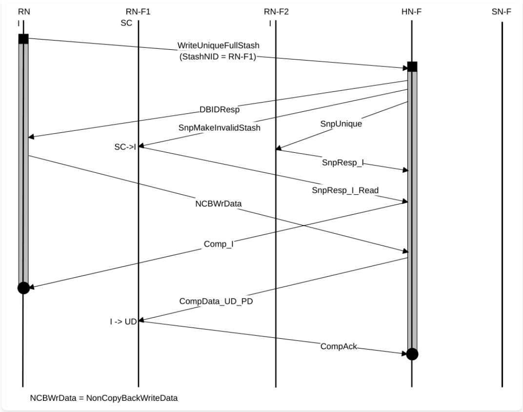
Figure p311 图 B5.23: 带 Data Pull 的 WriteUniqueFullStash
