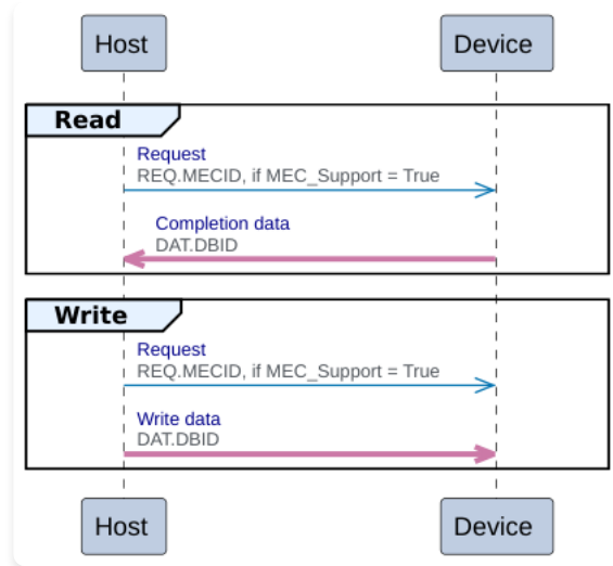
图 B10.3: 主机请求发往 DCM 位置时的 RME-CDA 字段
