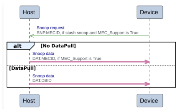
图 B10.4: 设备对已缓存 DCM 位置进行侦听时的 RME-CDA 字段
