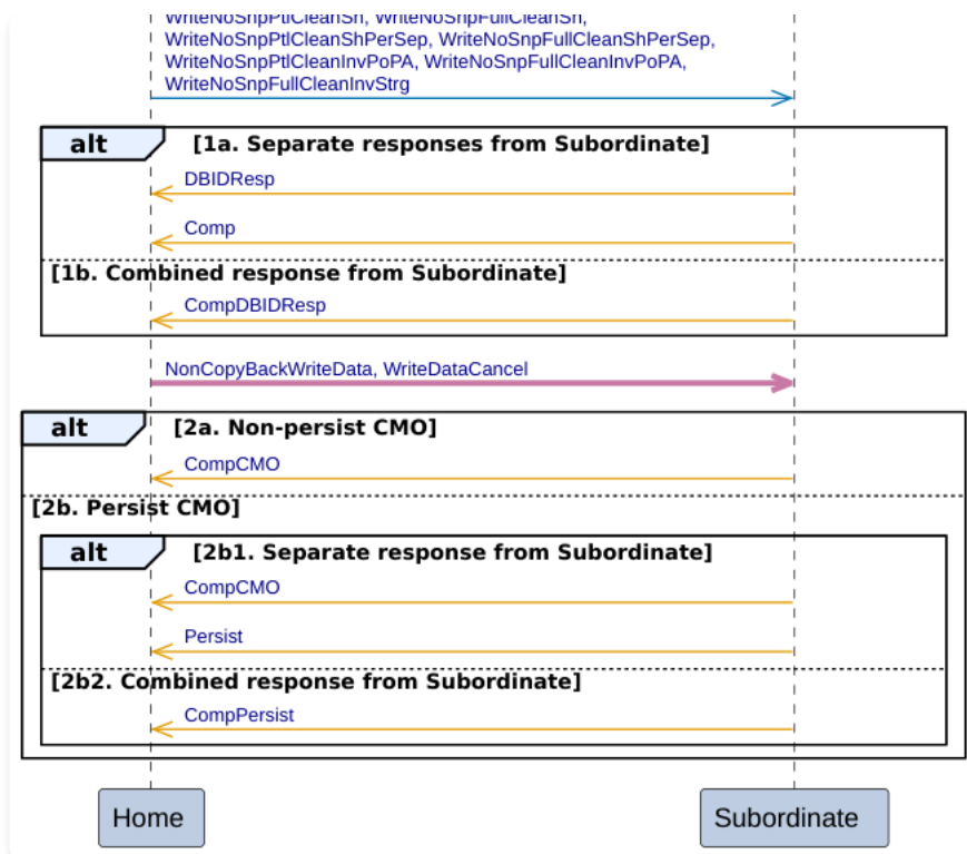
图 B2.18: 归属节点到从属节点的组合写与 CMO 事务
