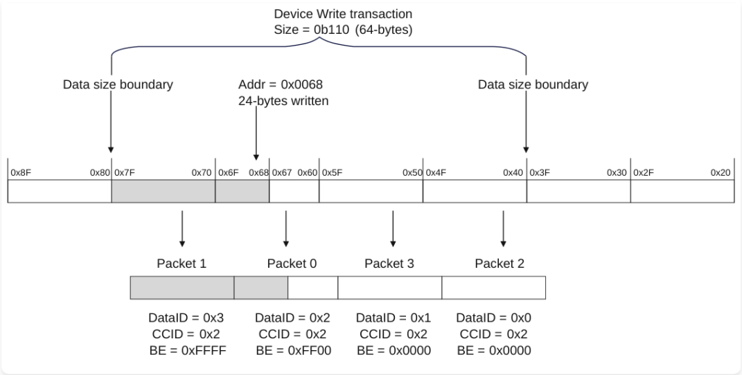
Figure p177 图 B2.49：发往非对齐地址的 Device 写事务
