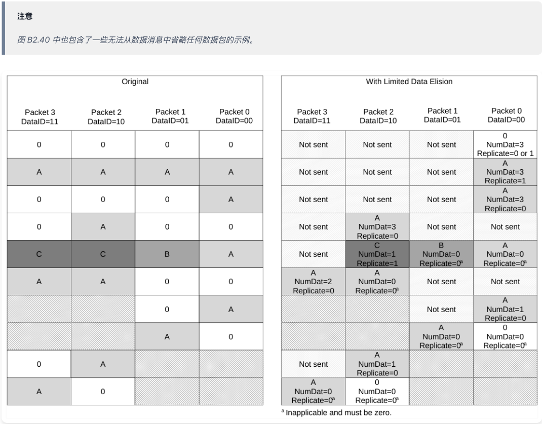
Figure p167 图 B2.40: 128 位数据总线宽度示例
