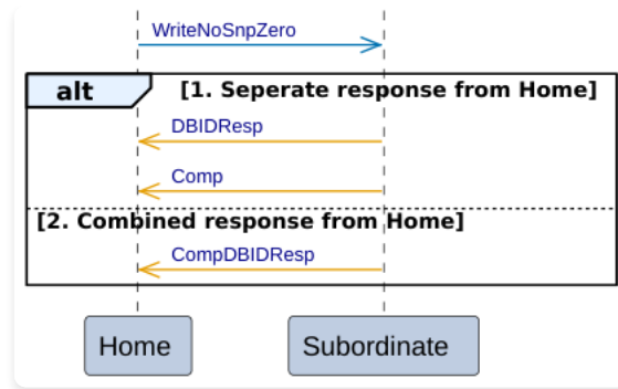
图 B2.17: 归属节点到从属节点的 Write Zero 事务
