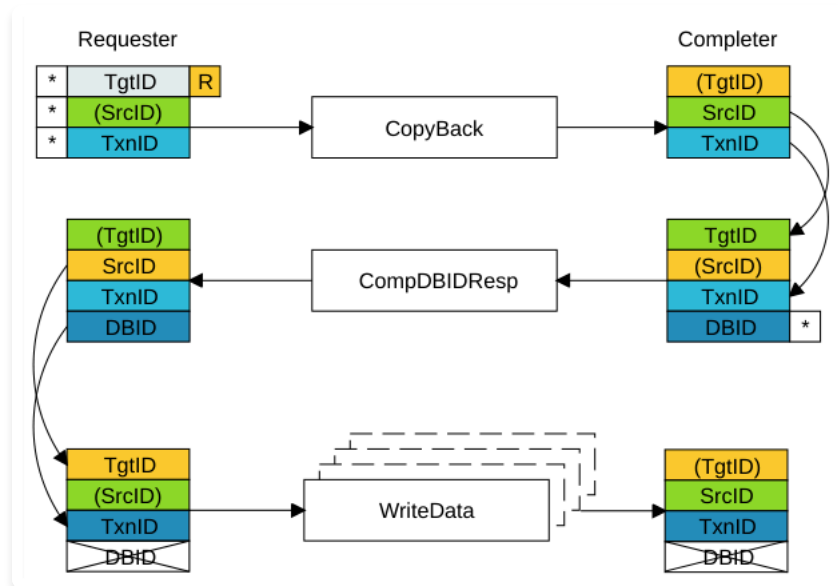
图 B2.28: CopyBack 中的 ID 值传递
