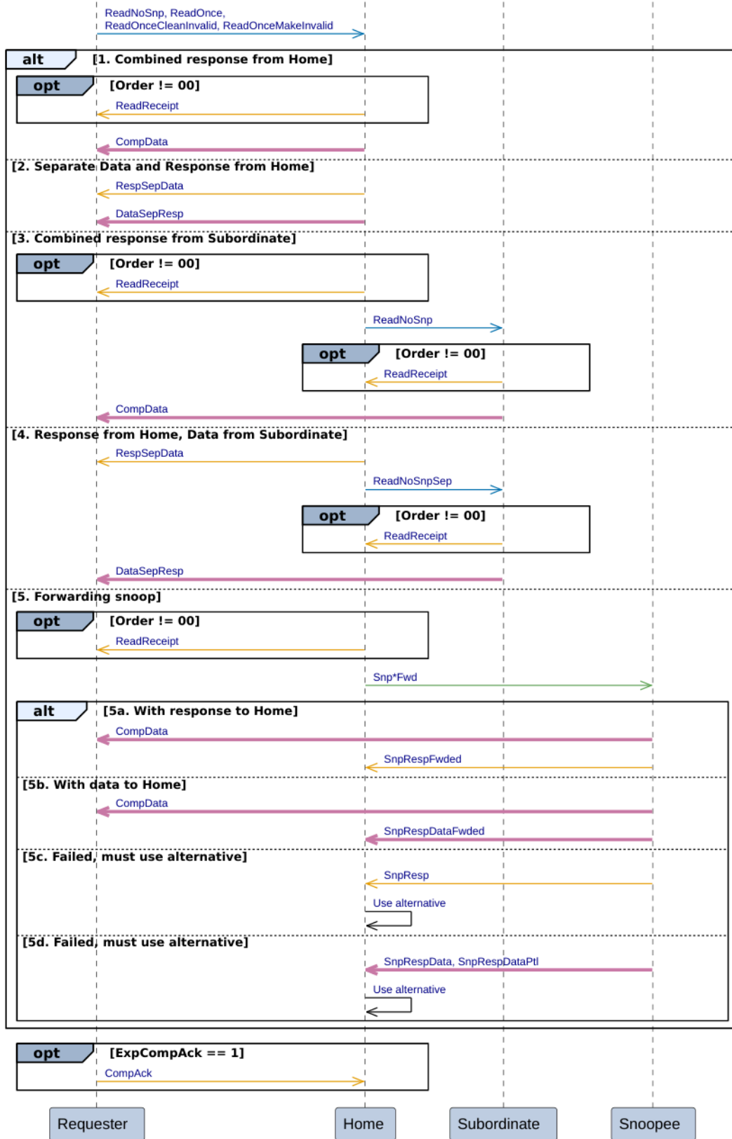
Figure p59 图 B2.2: 非分配读
