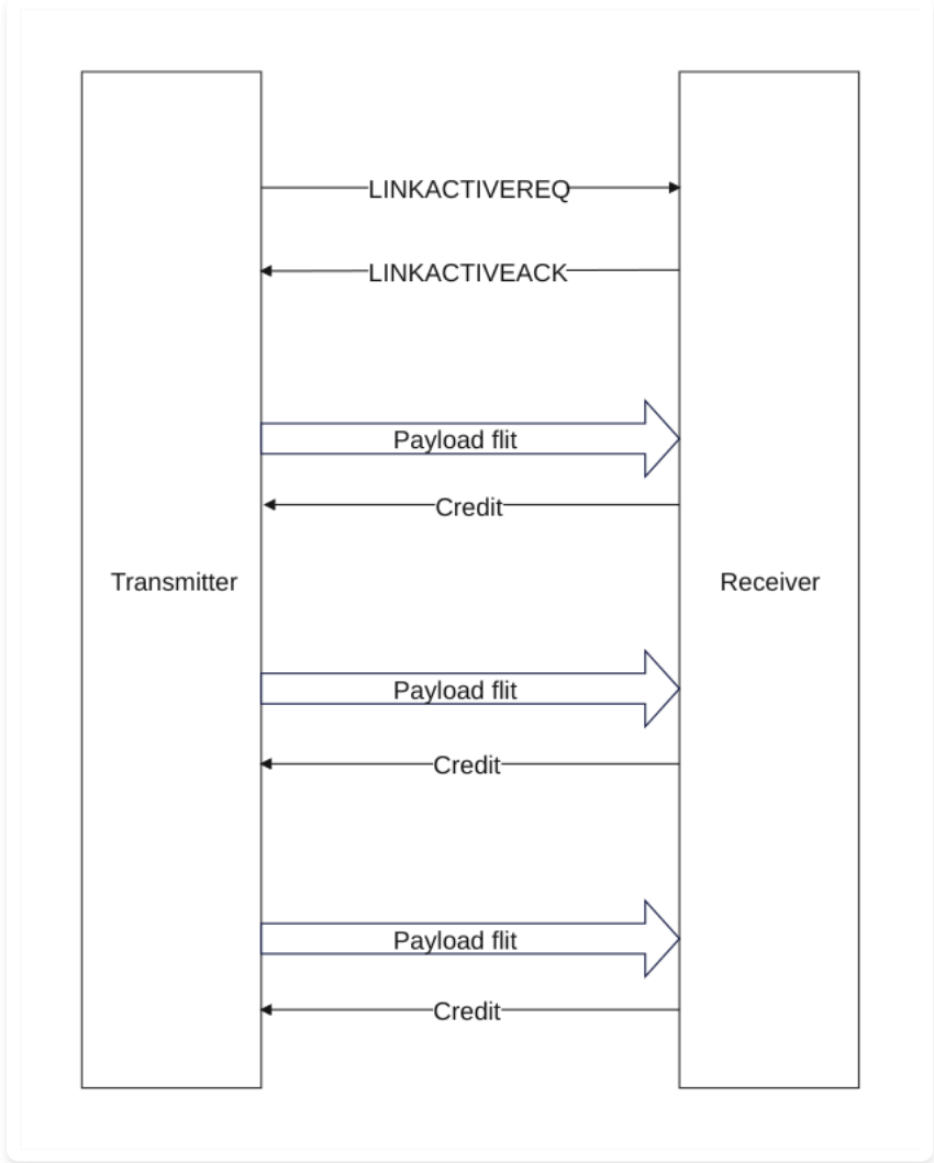
Figure p529 图 B14.6：多通道单向接口示例
