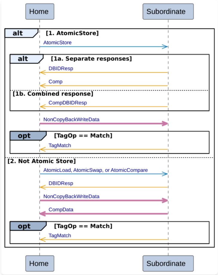
图 B2.20：归属节点到从属节点的 Atomic 事务
