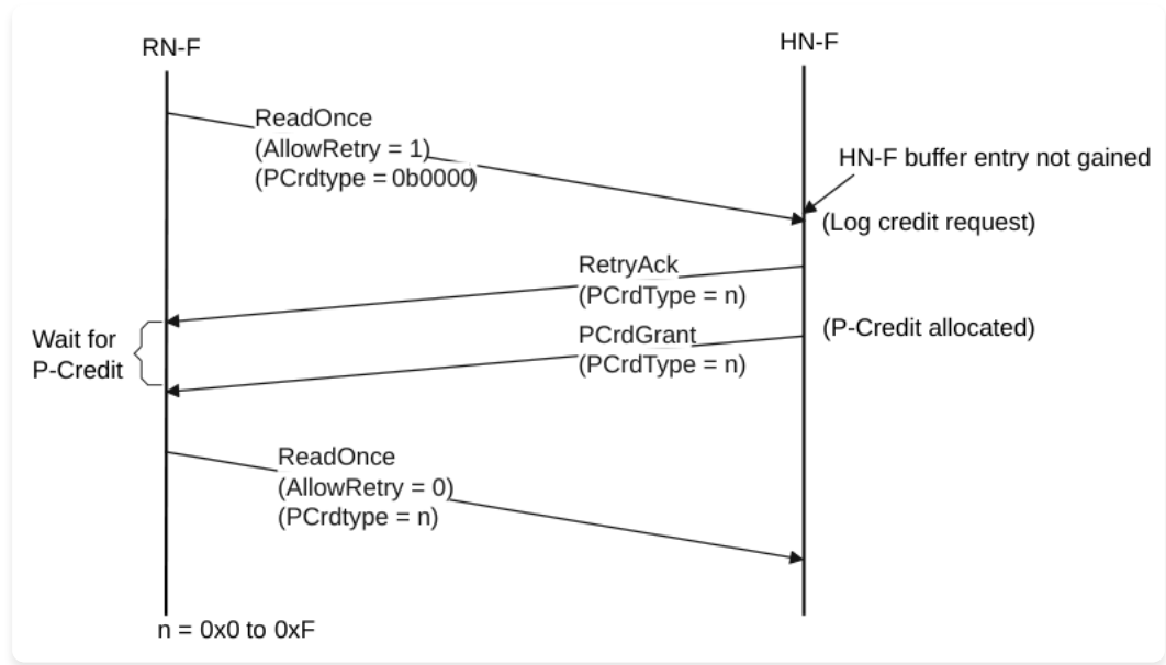
Figure p182 图 B2.50: Transaction Retry 流程
