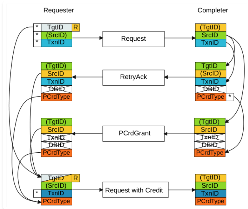
图 B2.33: 带 retry 的事务请求中的 ID 值传递
