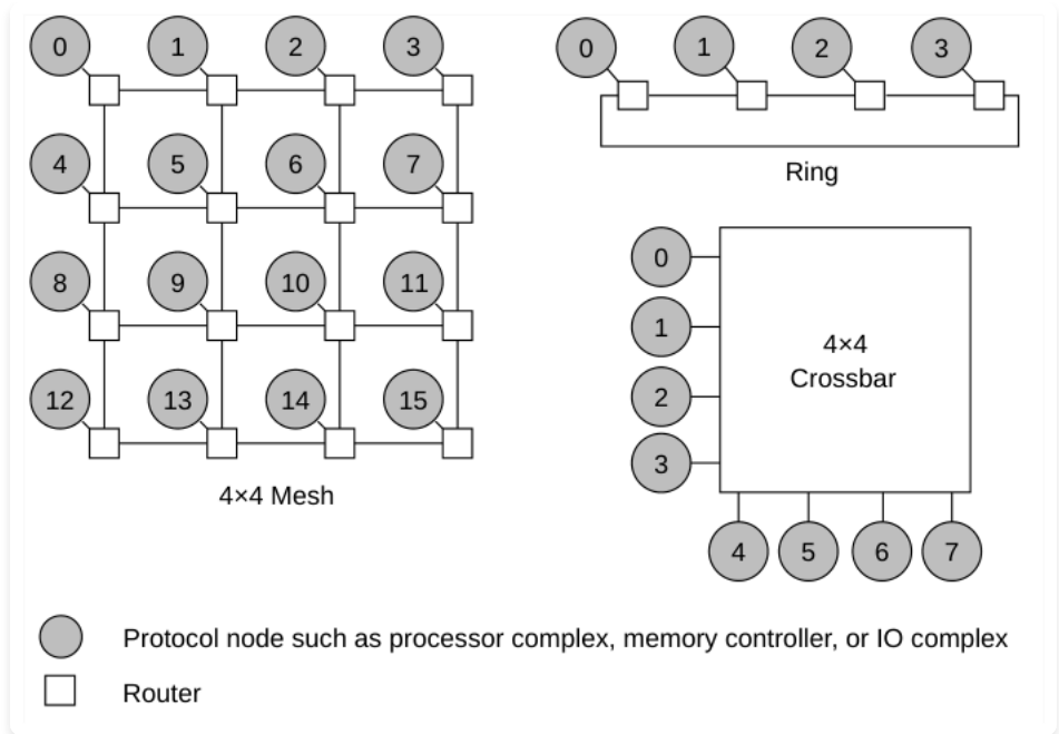
图 B1.1: 互连拓扑示例
