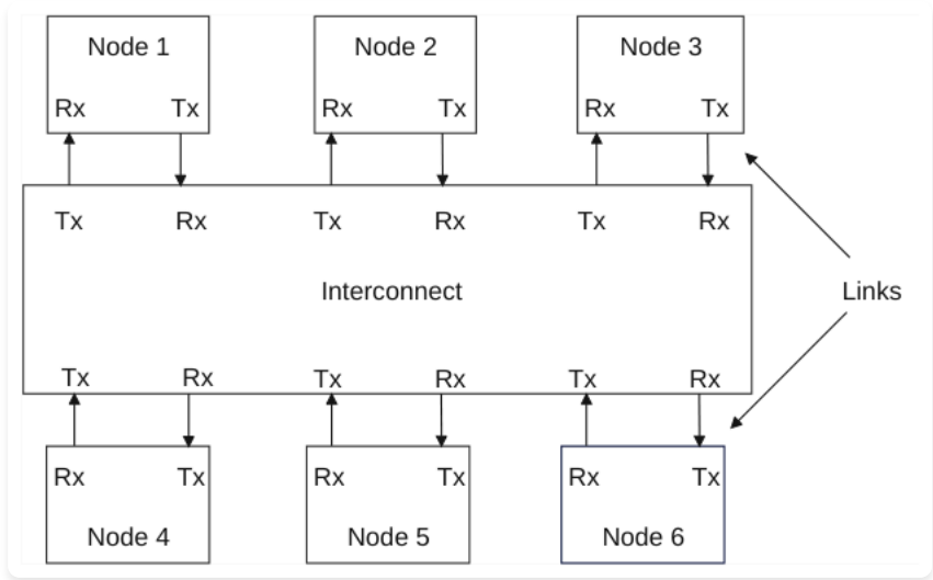
图 B13.1: 使用基于链路通信的系统
