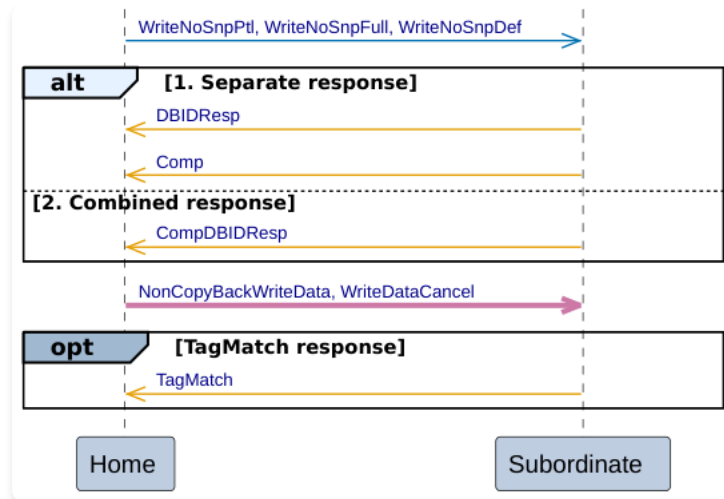
图 B2.16: 归属节点到从属节点写事务
