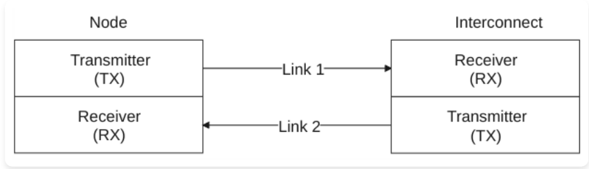
Figure p454 图 B13.2：双向链路通信
