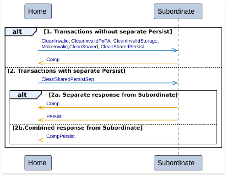
图 B2.19：归属节点到从属节点的 Dataless 事务
