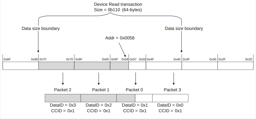
Figure p176 图 B2.48：来自非对齐地址的 Device 读事务
