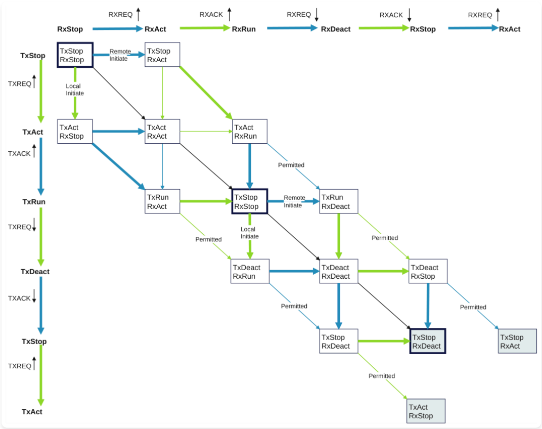
Figure p535 图 B14.9：无竞争条件的 Tx 与 Rx 组合状态机
