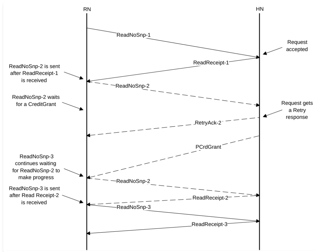
图 B2.38：一系列有序读请求
