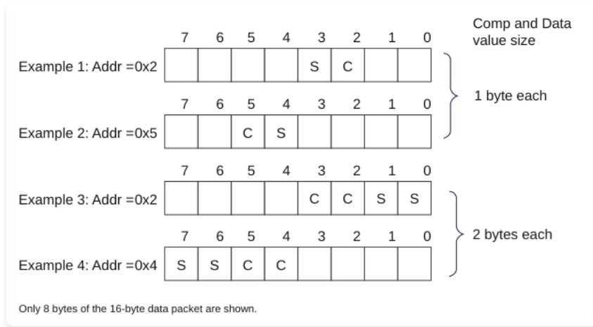
图 B2.43: AtomicCompare 事务的数据值打包
