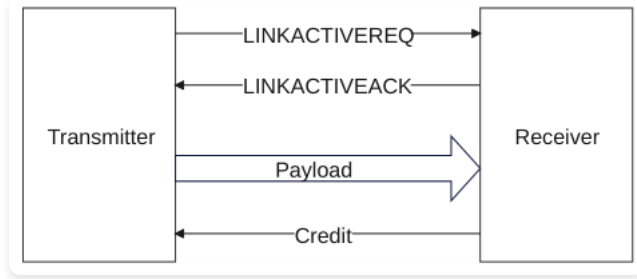
图 B14.4: Payload、Credit 与 LINKACTIVE 信号之间的关系
