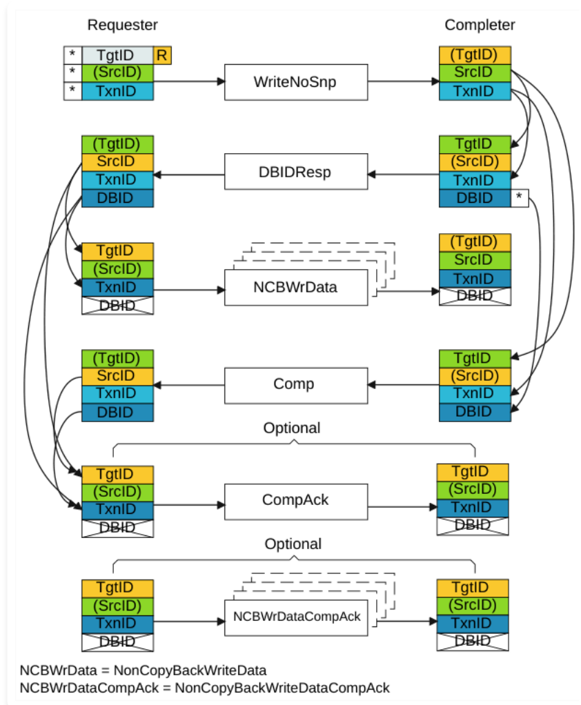
图 B2.29: WriteNoSnp 中的 ID 值传递
