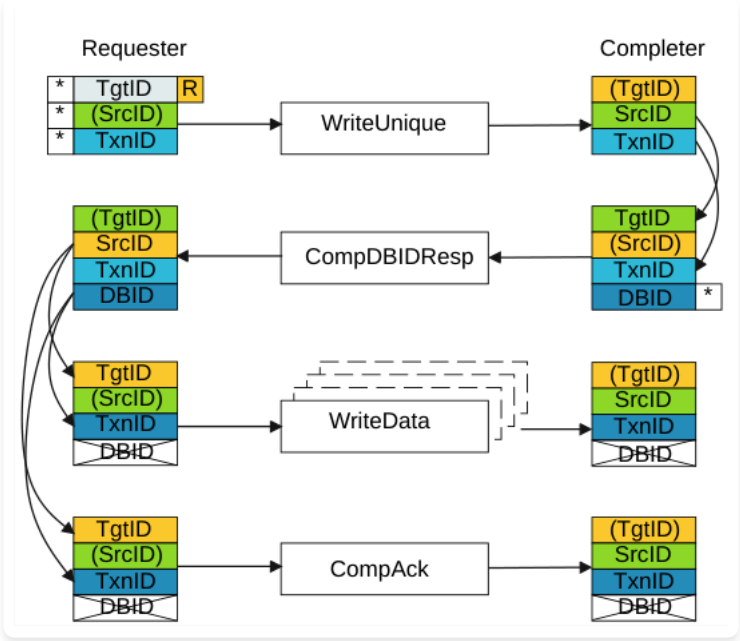
图 B2.30: 使用合并的 CompDBIDResp 响应时的 ID 值传输
