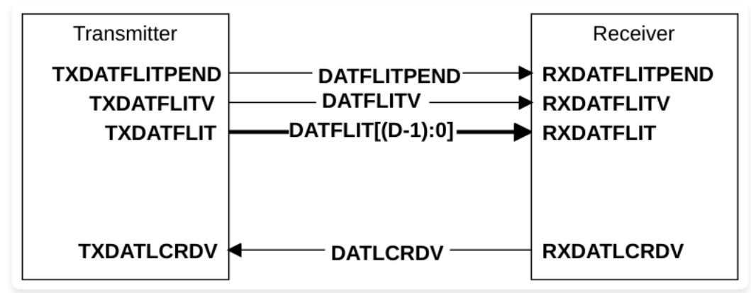
Figure p469 图 B13.14：DAT 通道接口引脚
