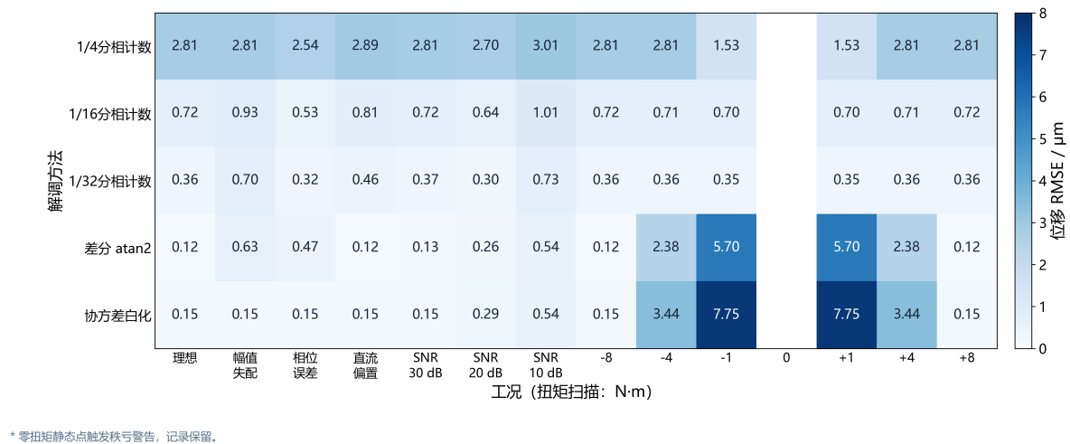
图 6 14 类工况下五种解调算法的位移 RMSE 热图
