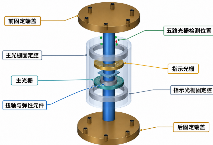
图 2 光栅扭矩测量机械—光学结构示意图
